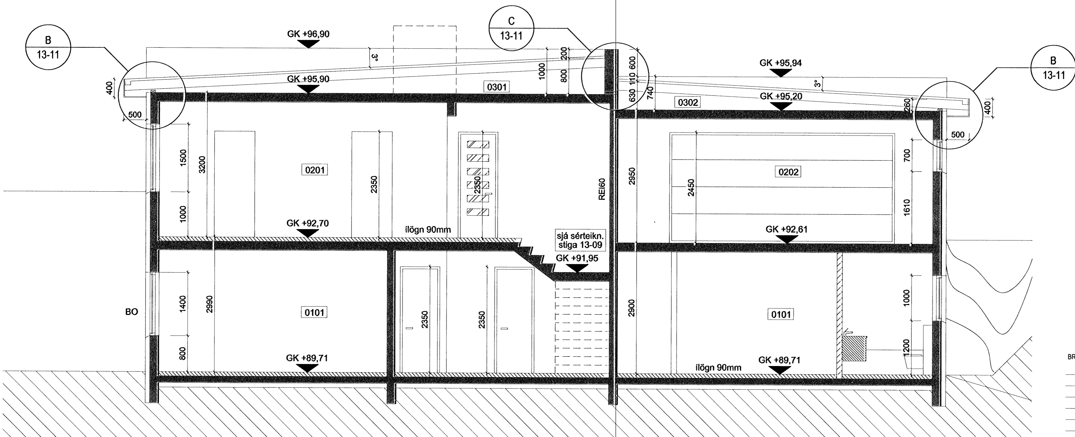
SNEIÐING X-X 1:50
