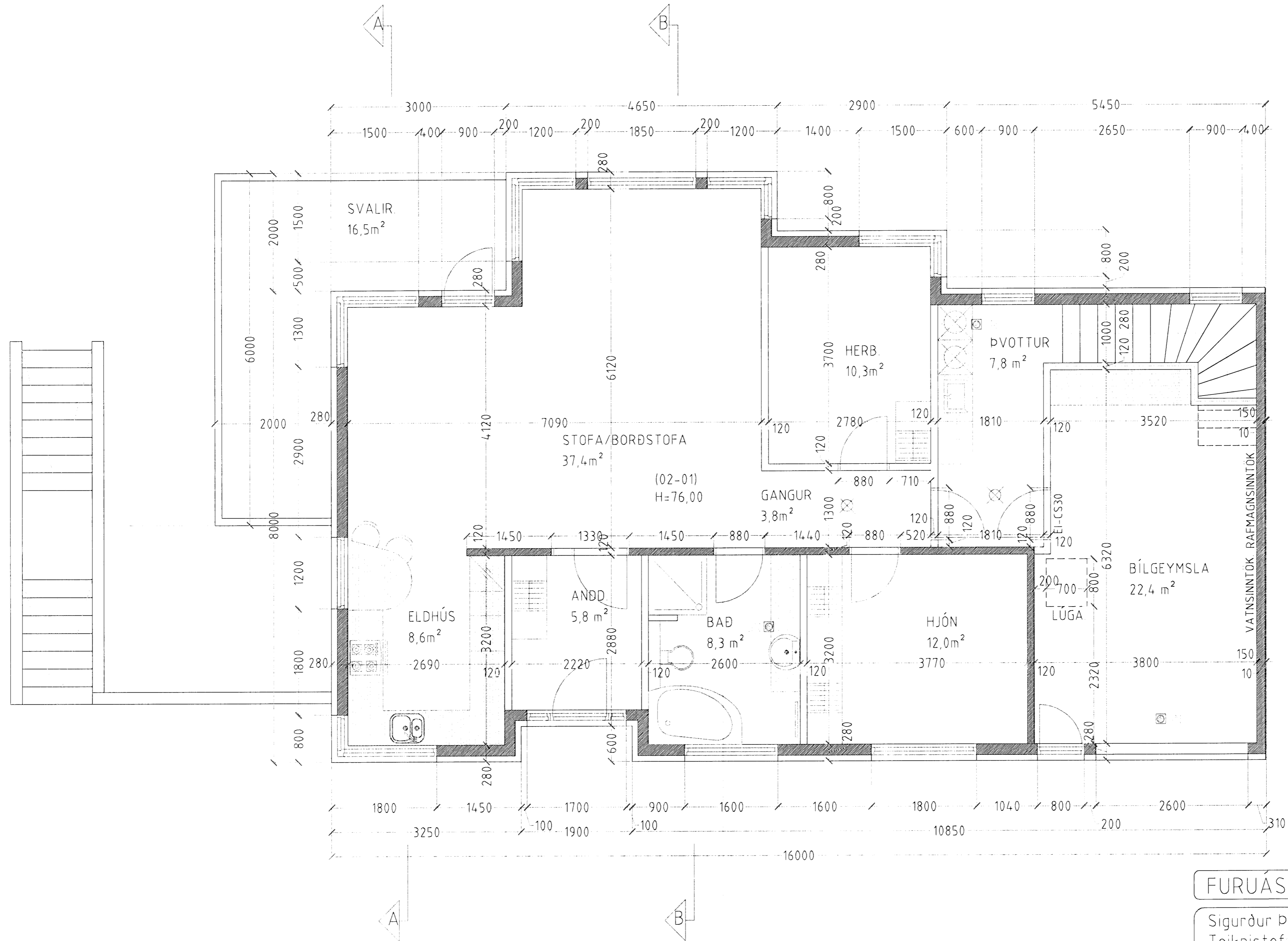
GRUNNMYND 1. HÆÐ MKV. 1:50.
