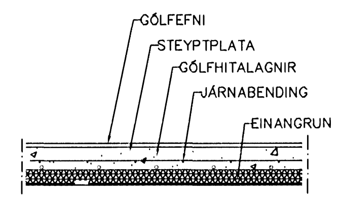
LAGNIR, SNÍÐ, 1:20
