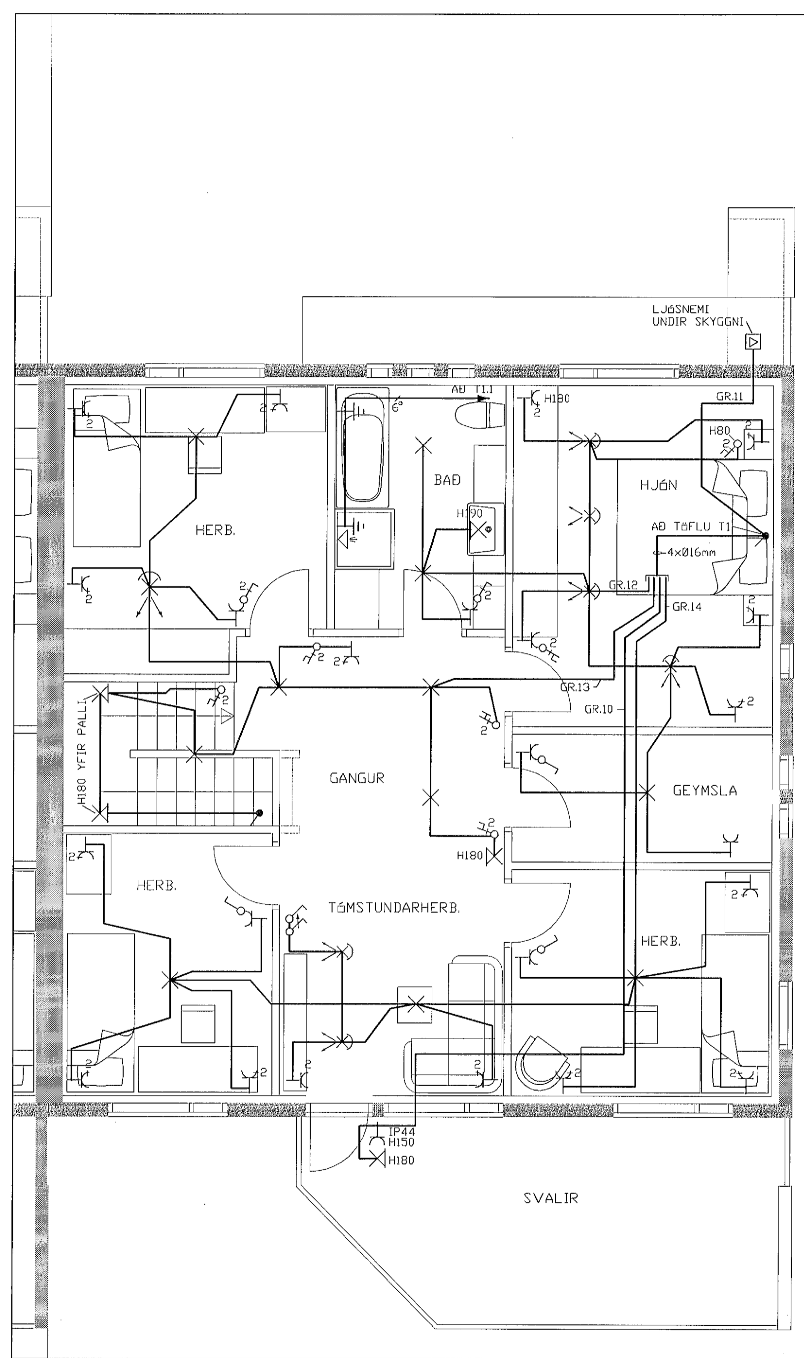
GRUNNMYND 2. HÆÐ
