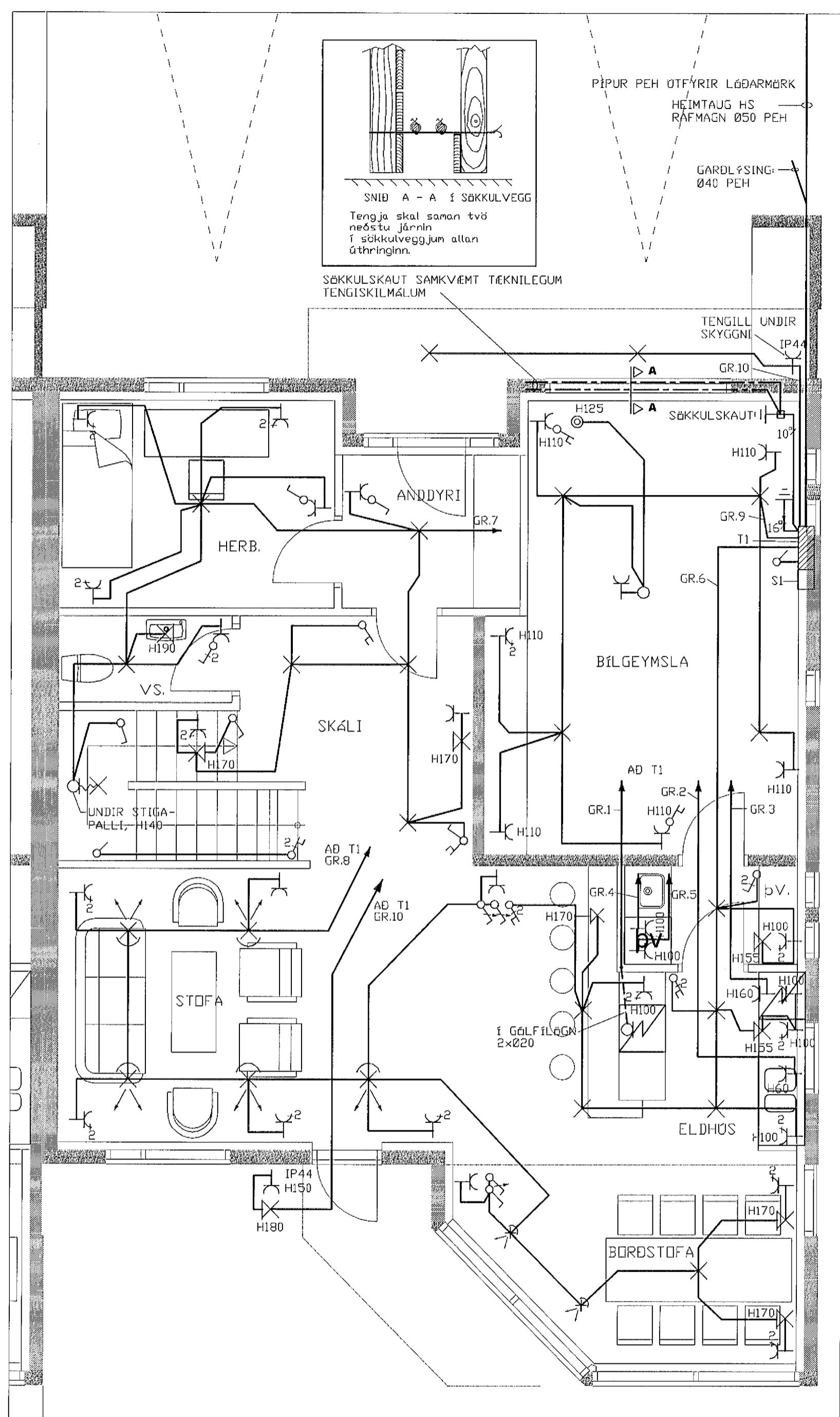
GRUNNMYND 1. HÆÐ
