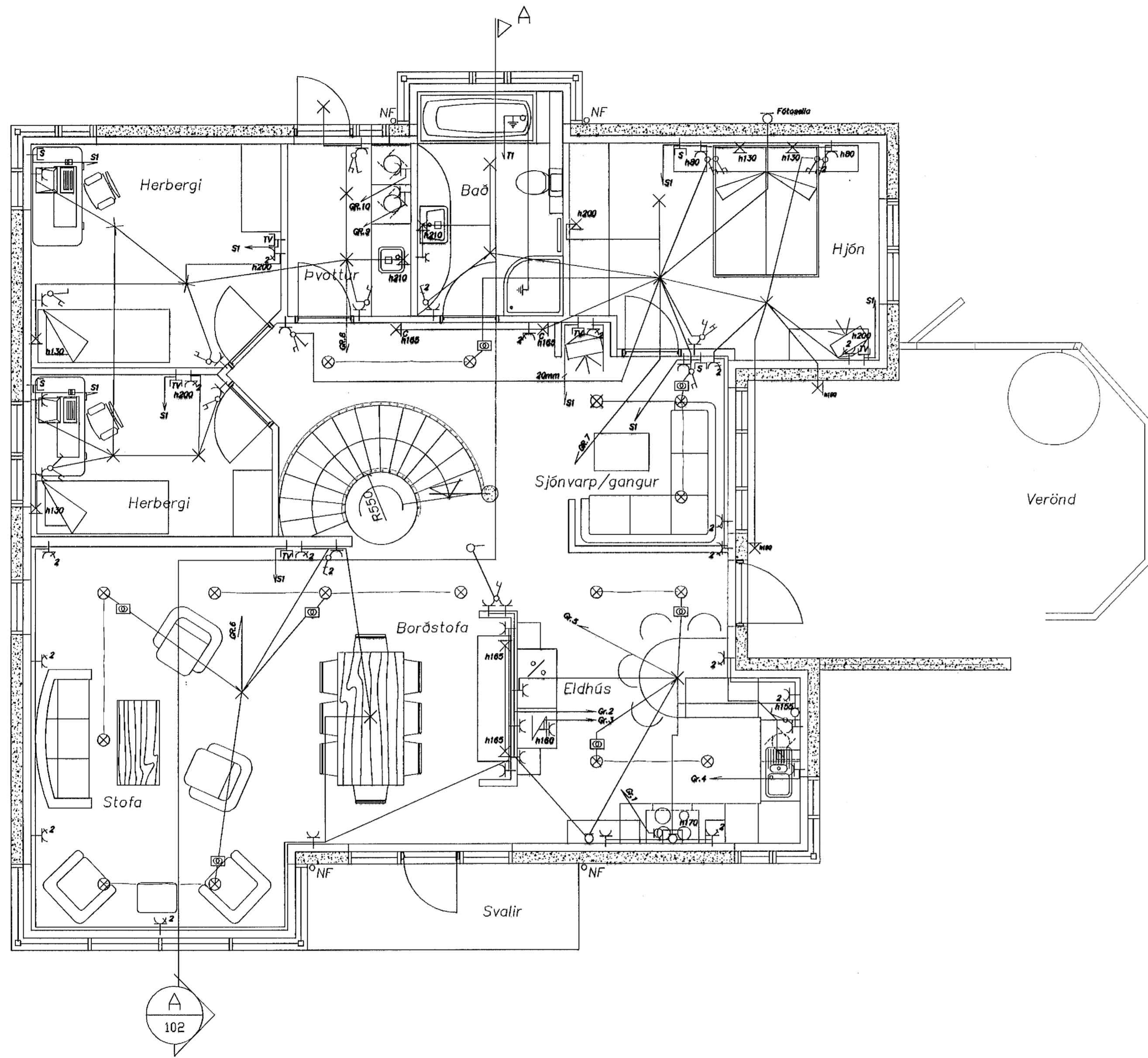
Grunnmynd, aðalhöðar Mælikvarði 1:50
