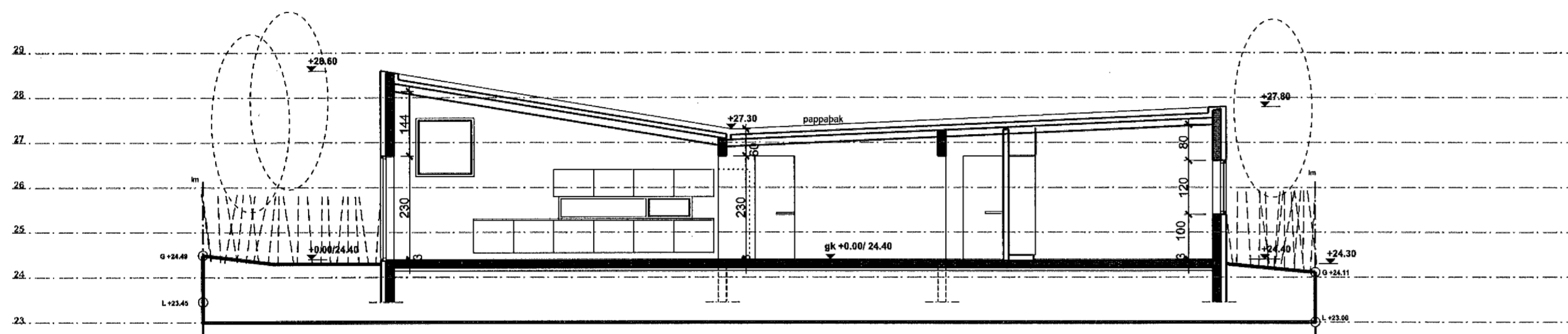
SKURÐMYND A-A
