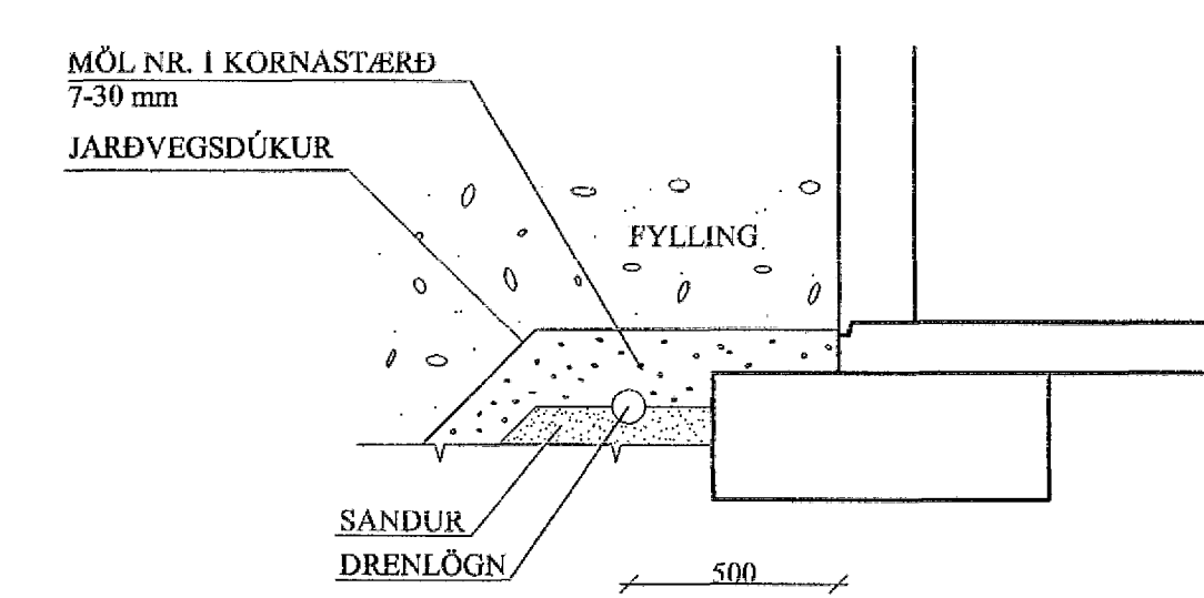
DRENLOGN KENNISNIÐ 1:20
