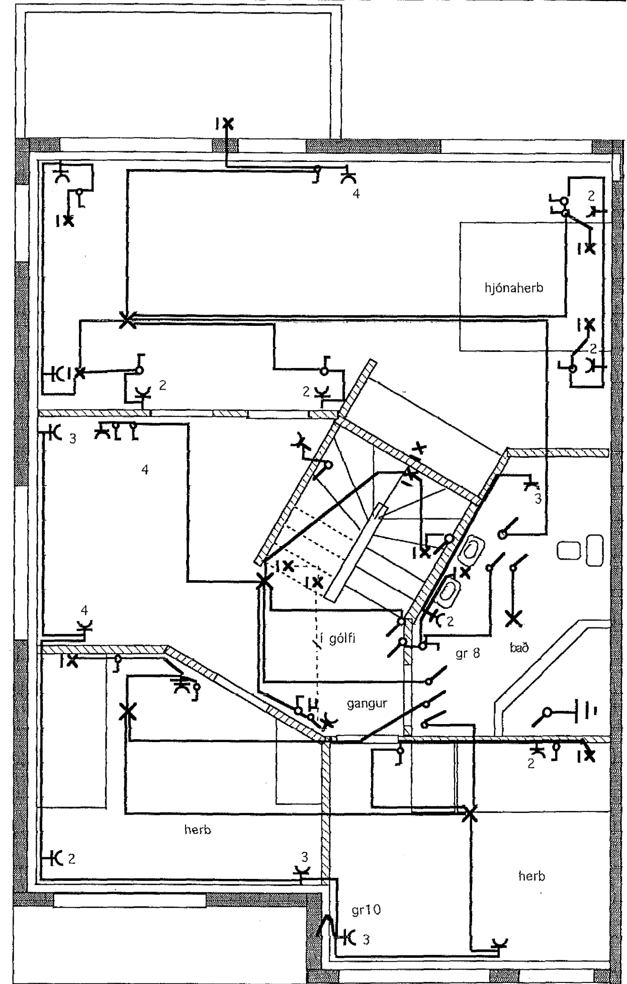
Tinnuberg 12 Raflögn. Teiknari Jónas Stefánsson. MKV 1:50 teiknað júní 1994.
