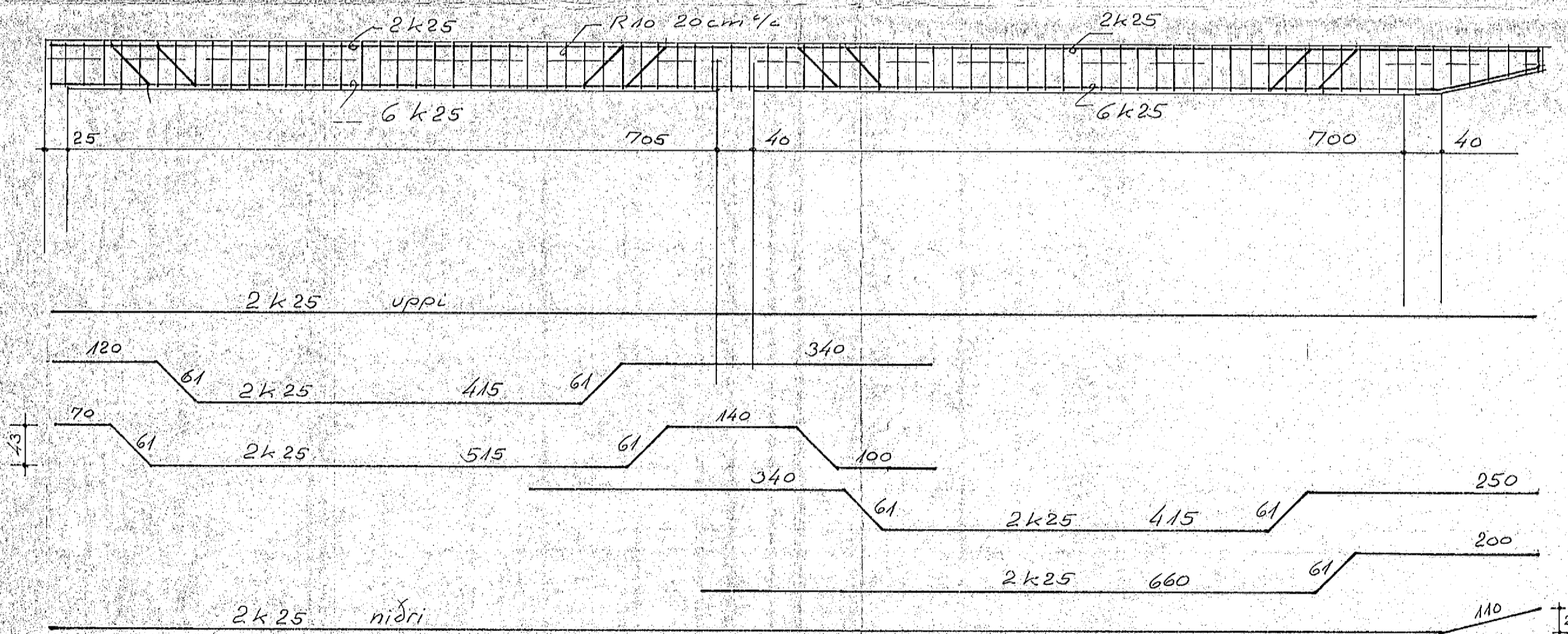
Langsnið 1:20
