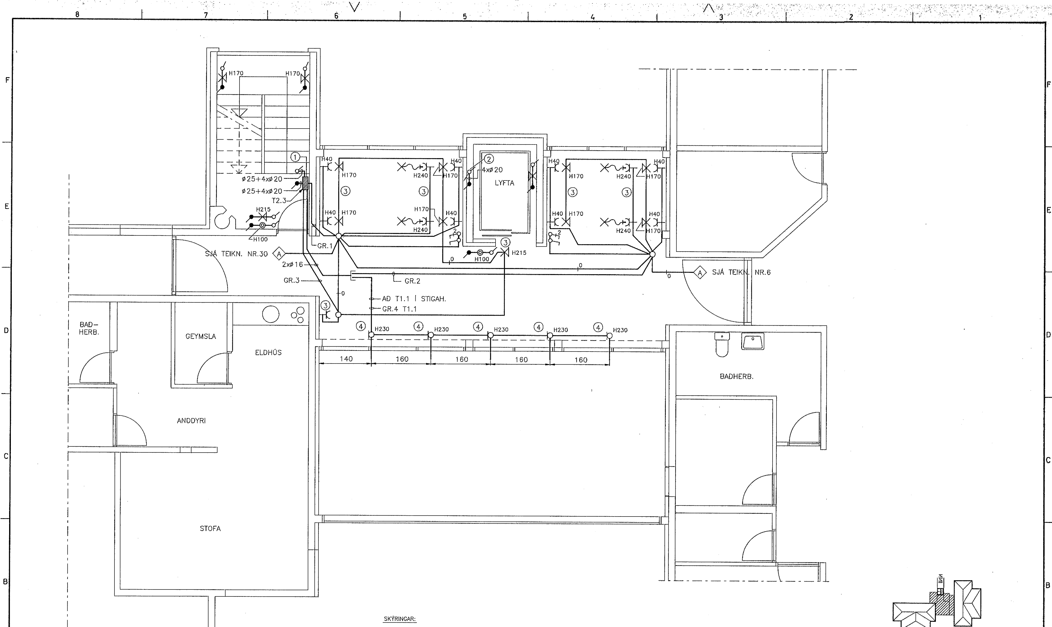
GRUNNMYND 2.HÆÐ TENGBYGGING MKV: 1:50
