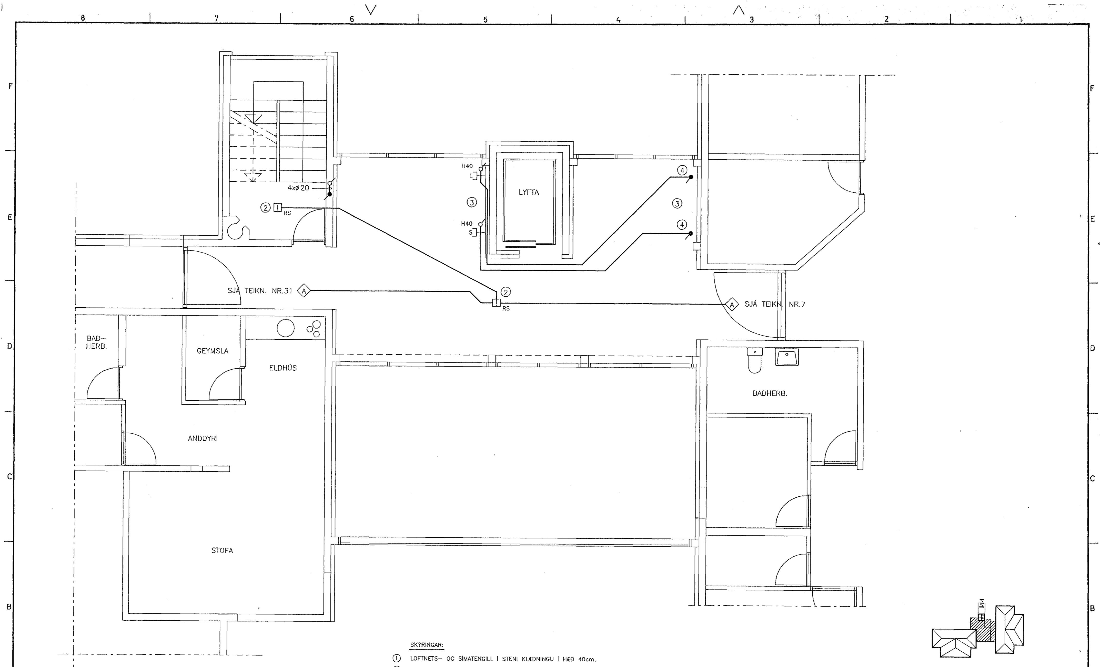
GRUNNMYND 2.HÆÐ TENGBYGGING MKV: 1:50
