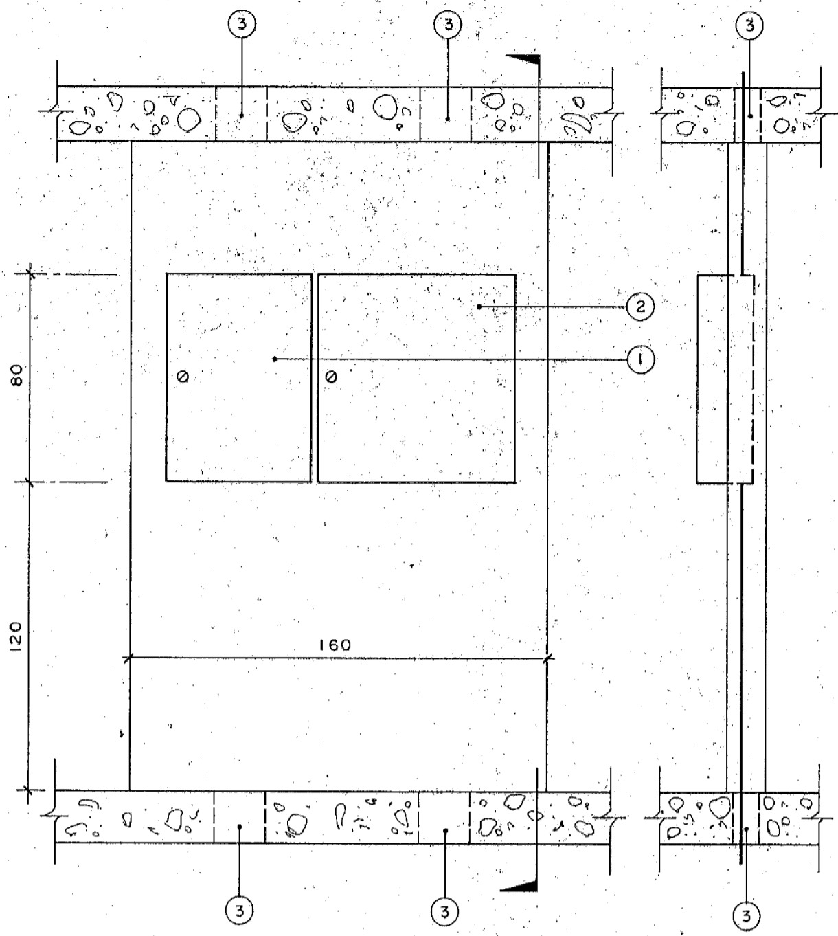
A SNIÐ M. 1:20 41 | 44
