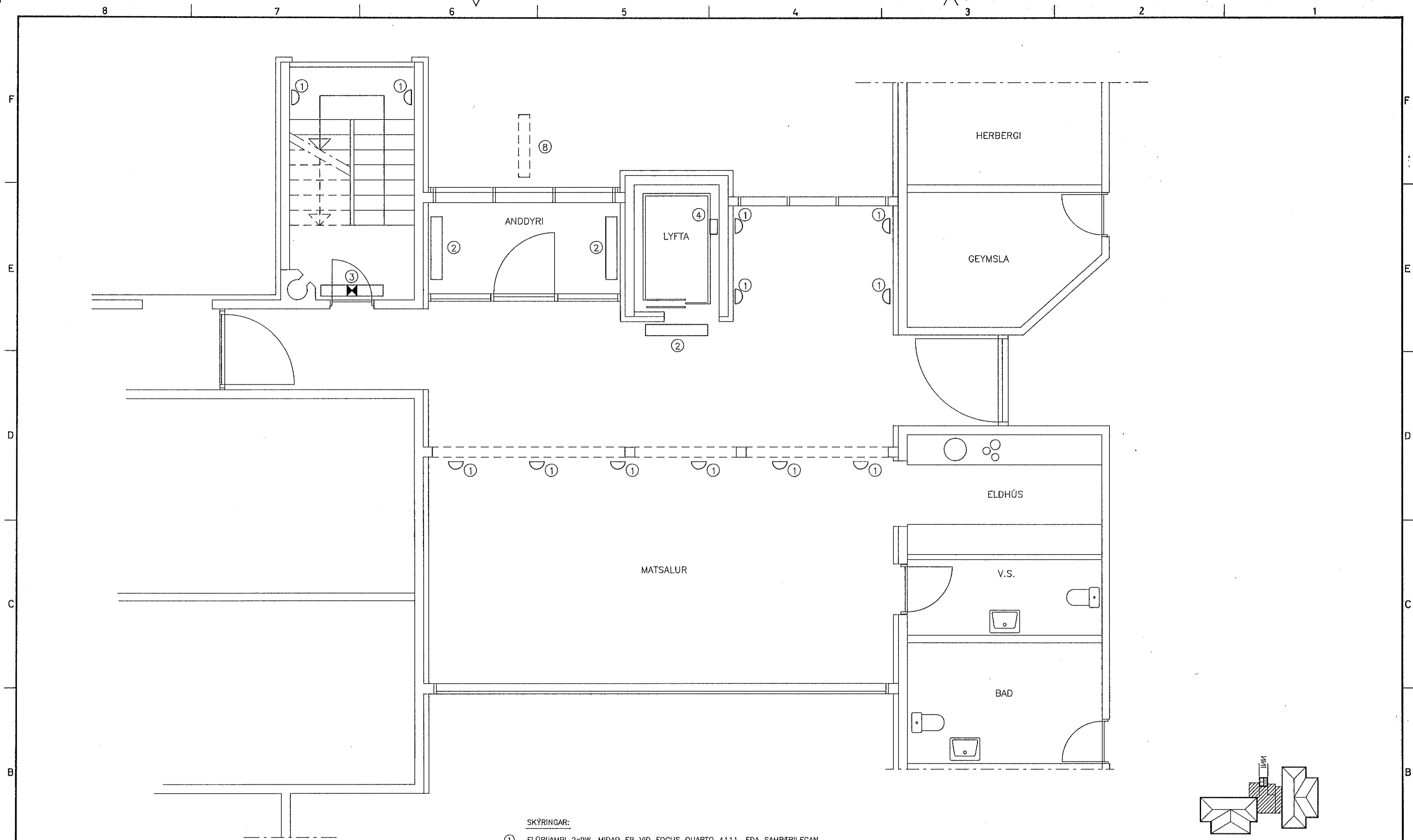
GRUNNMYND 1.HÆÐ TENGIÞYGGING MKV: 1:50
