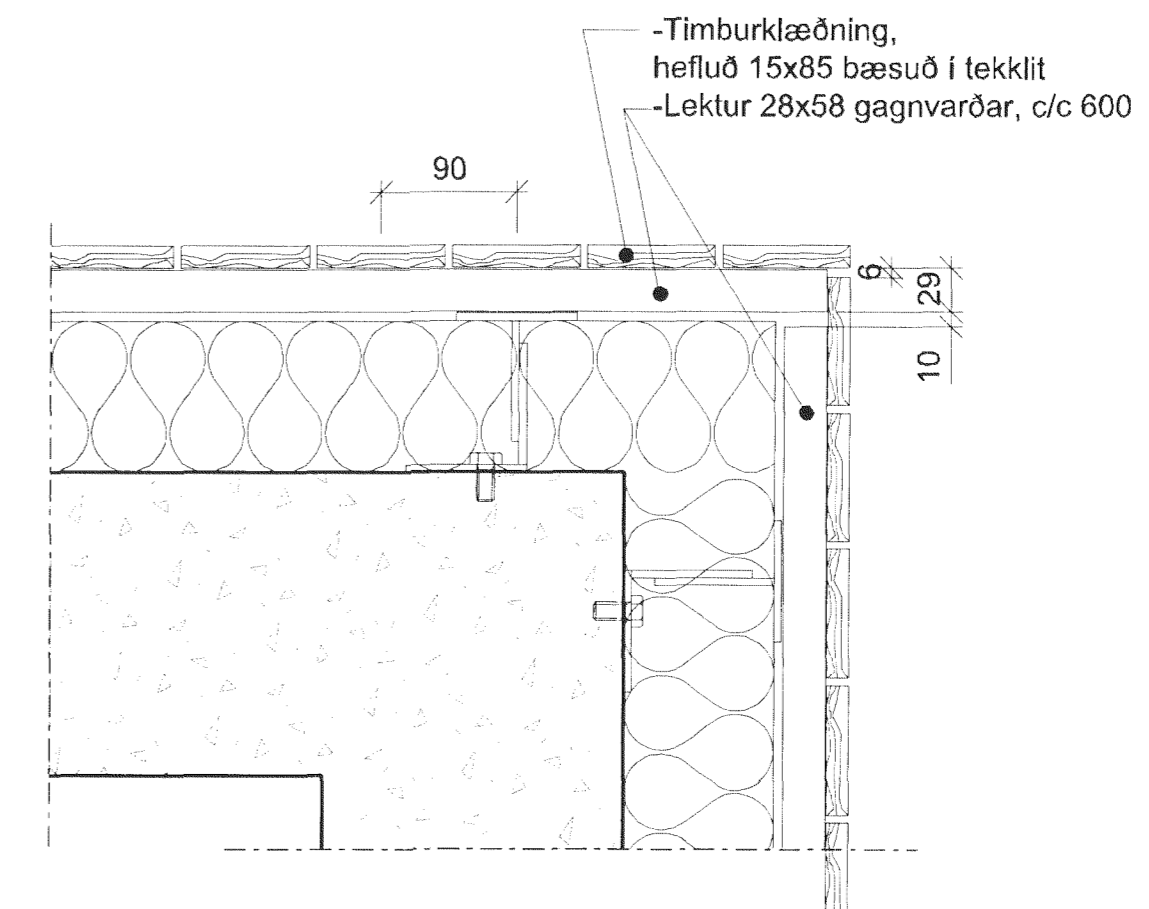
8 DEILI 1:5 ÚTHORN, VIÐUR/VIÐUR
