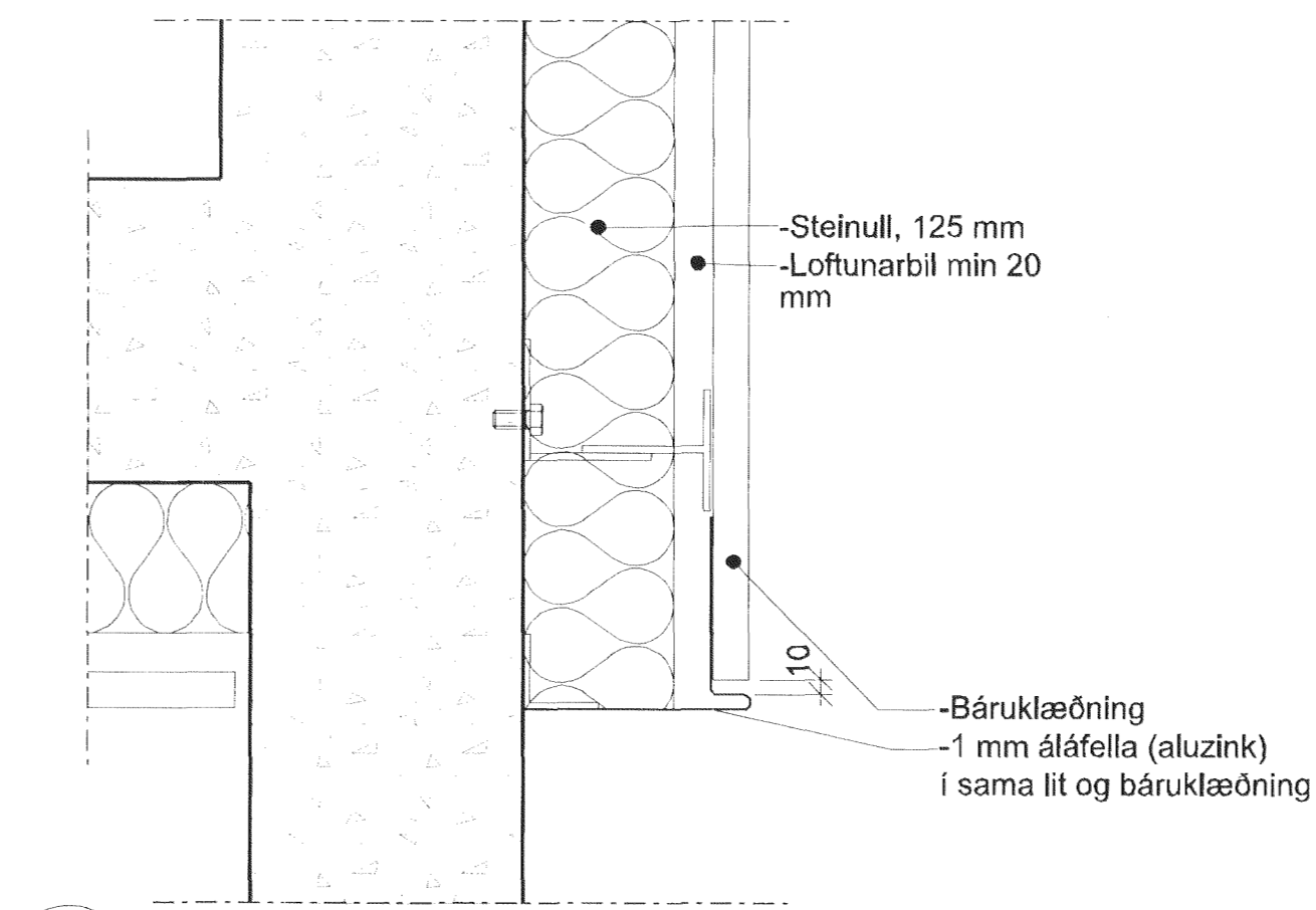
11 DEILI 1:5 BÁRA, LOKUN Á EINANGRUN
