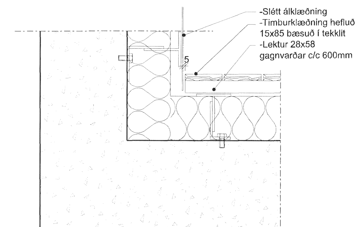
4 DEILI 1:5 INNHORN, SLÉTT/VIÐUR
