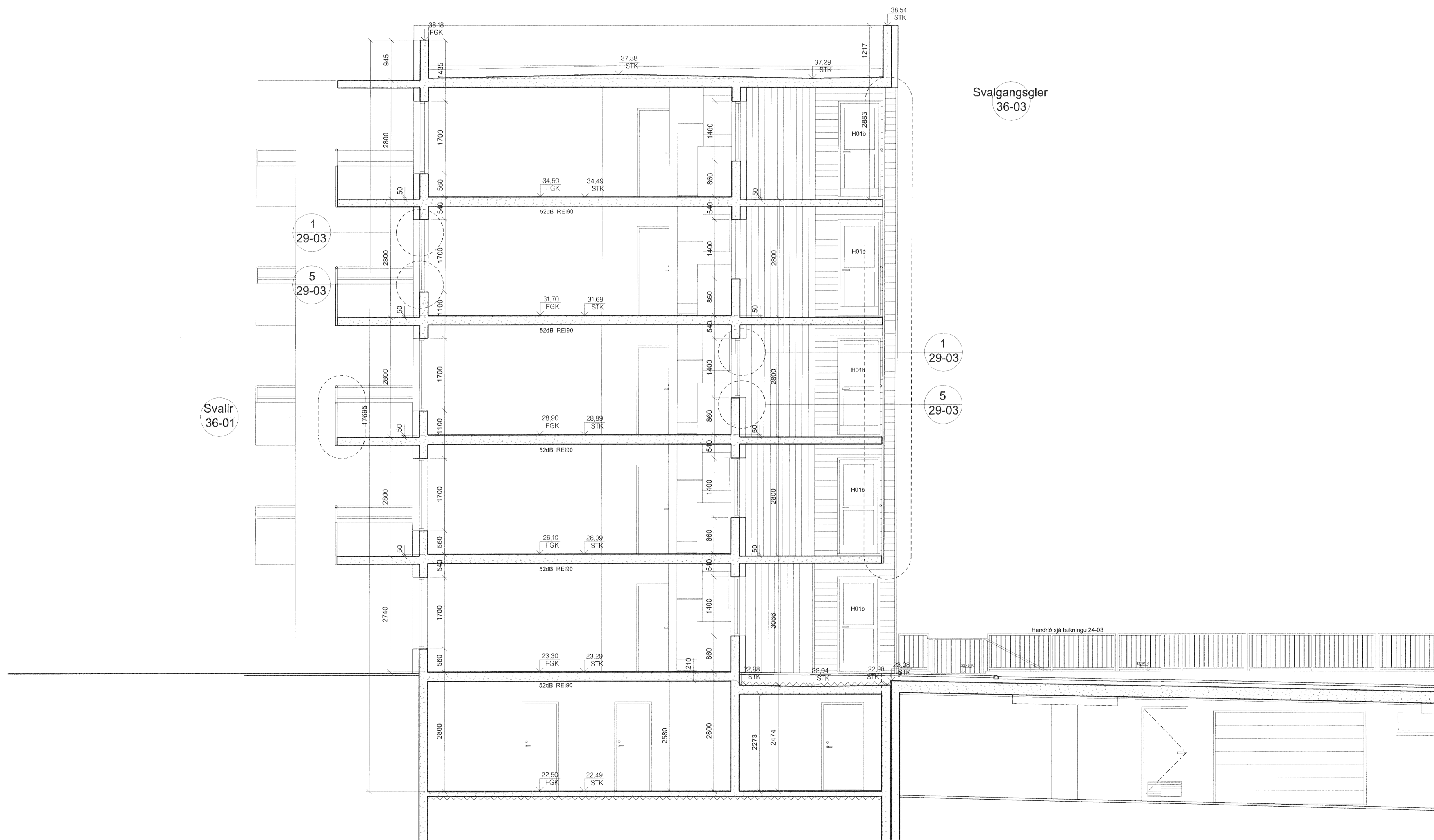
H-H 20-01 20-03 20-05 20-07 20-09 20-11 20-13 SNEIÐING 1:50
