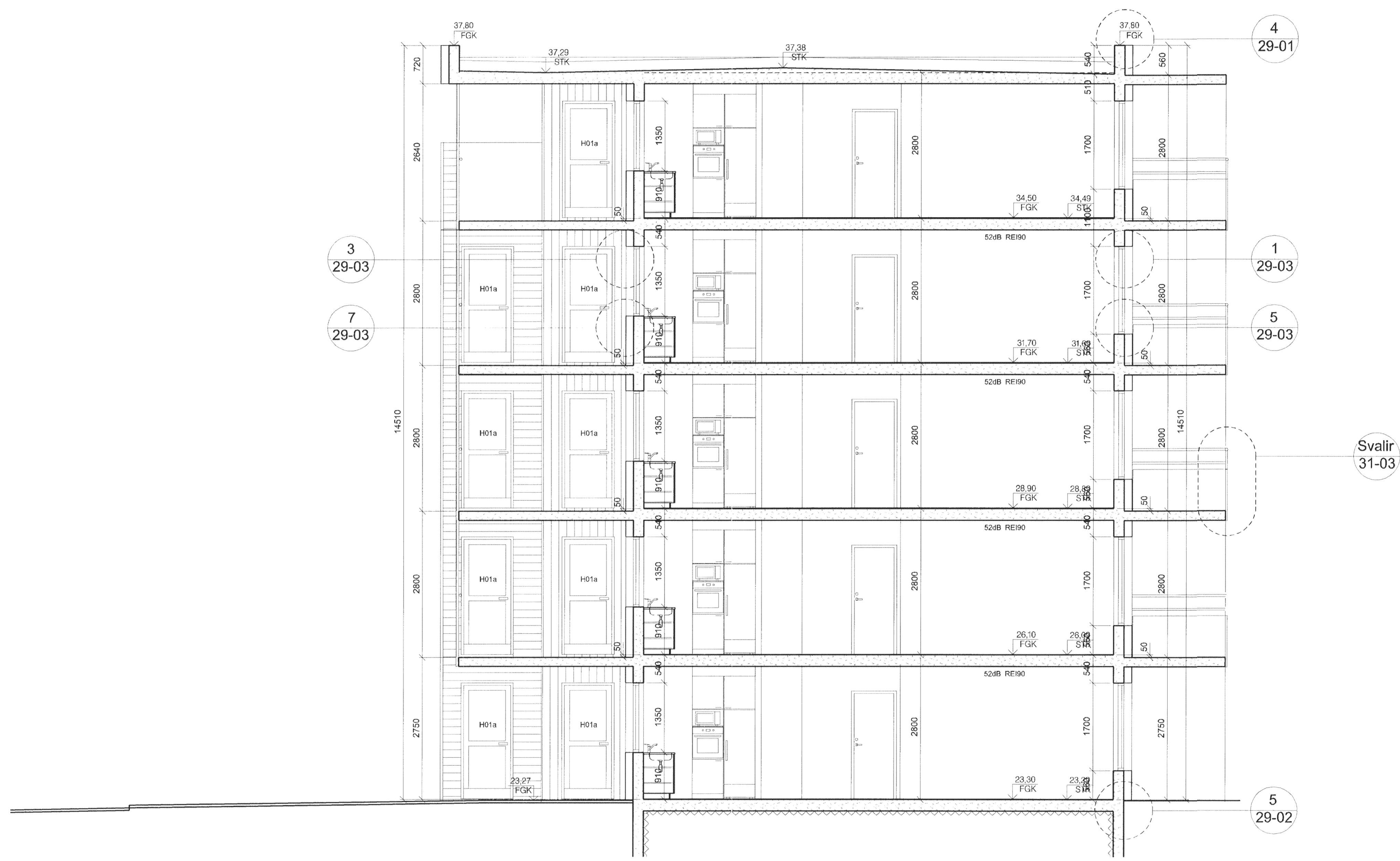
G-G 20-02 20-04 20-06 20-08 20-10 20-12 20-14 SNEIÐING 1:50
