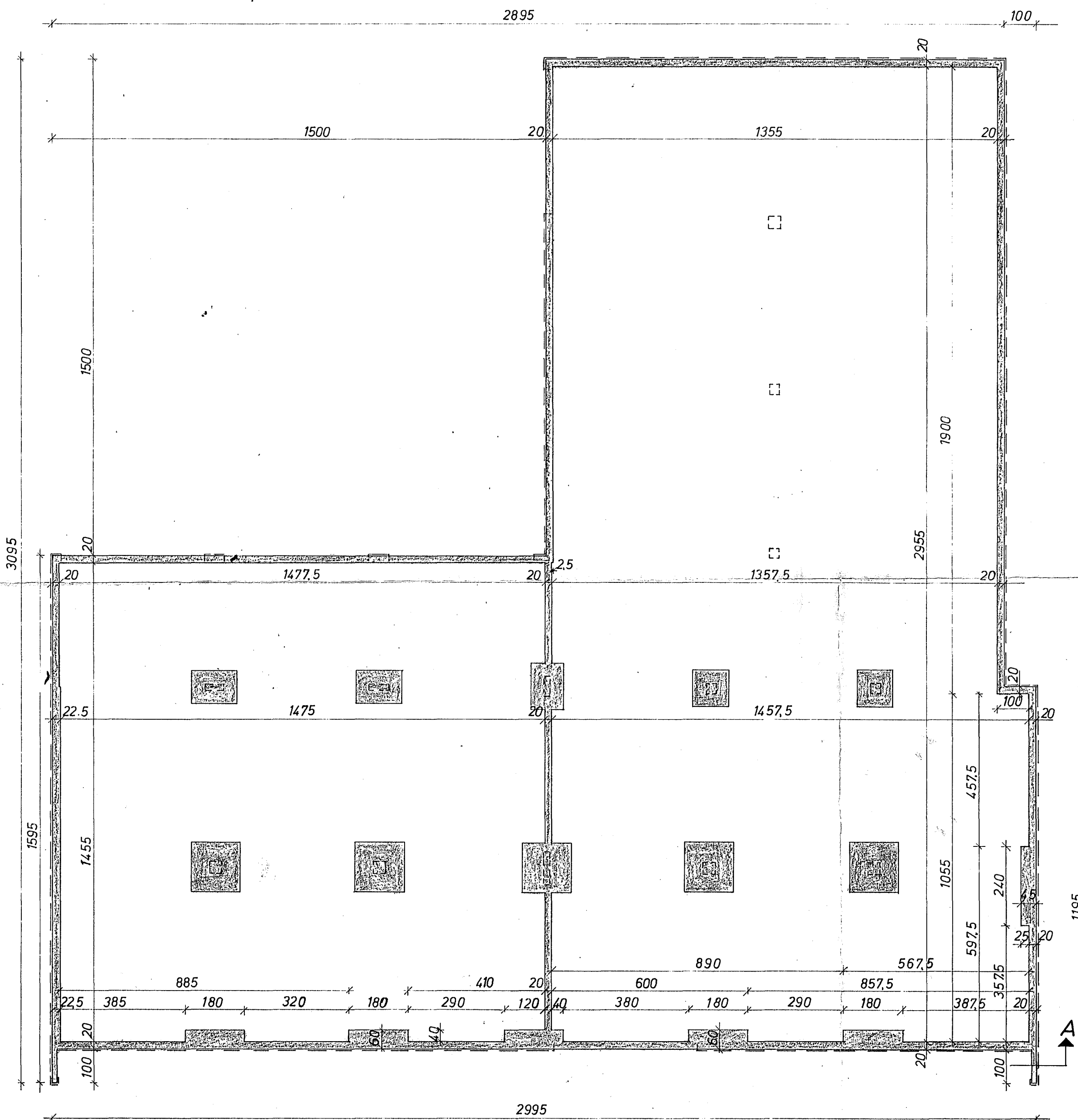
GRUNNMYND 1:100
