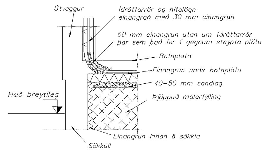
D Kennisnið við útvegg Málkvörði 1:20
