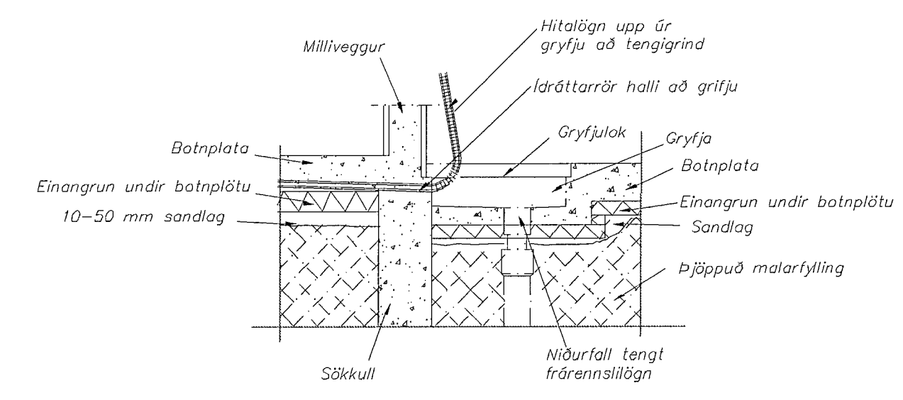
B Snið í gryfju við tengigrind Málkvörði 1:20
