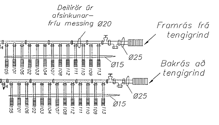
B Deili - Tengimynd dreifingar Málkvörði 1:20
