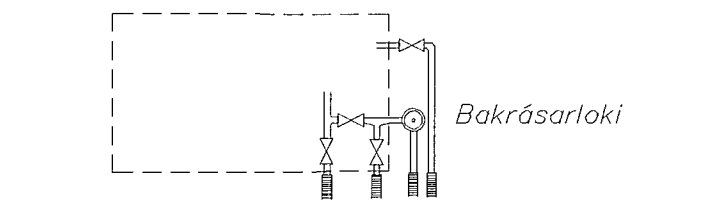
C Kennisnið tengingar bakrásar frá ofnum við gólflita Málkvörði 1:20
