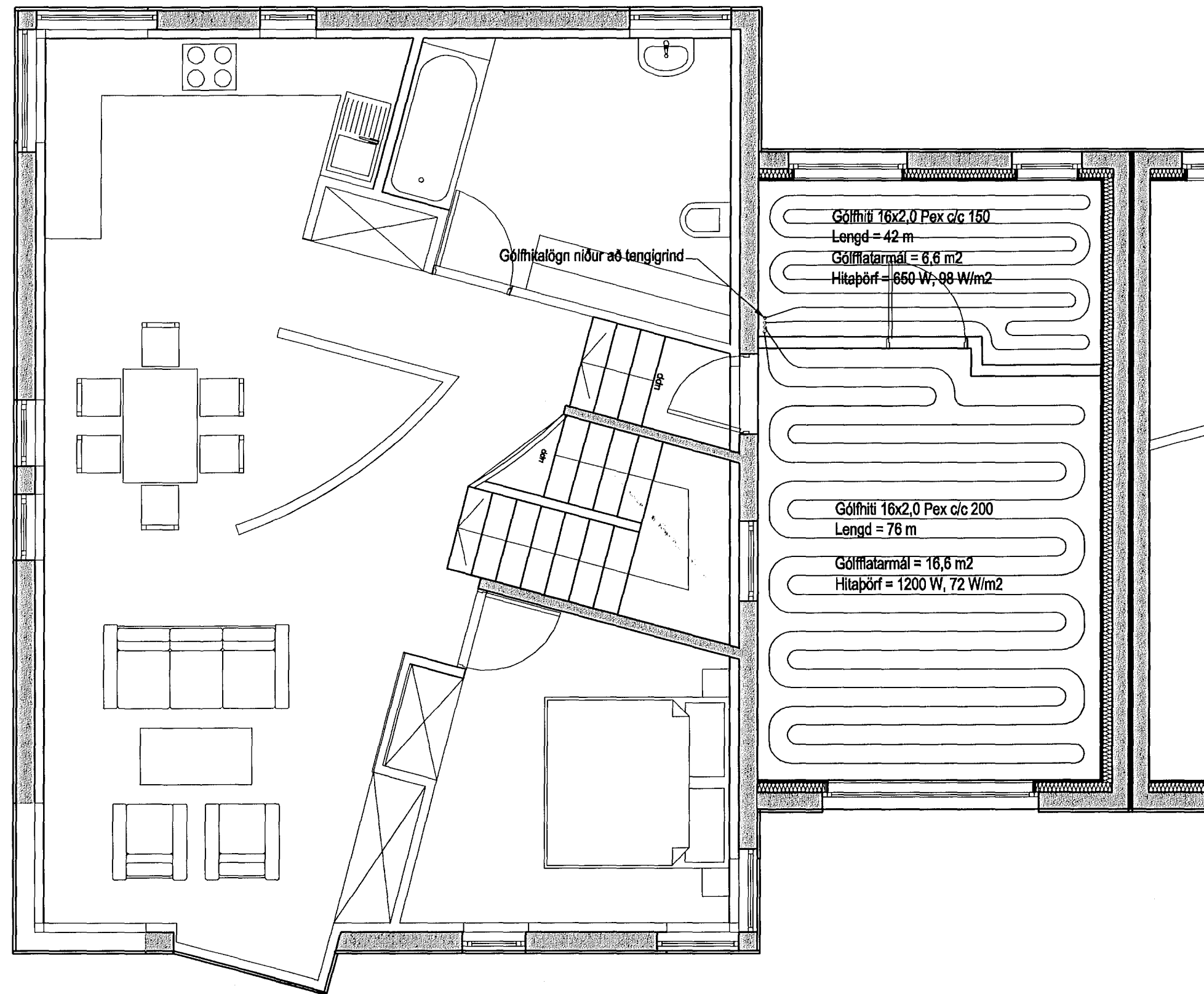
2. hæð, Grunnmynd, 1:50
