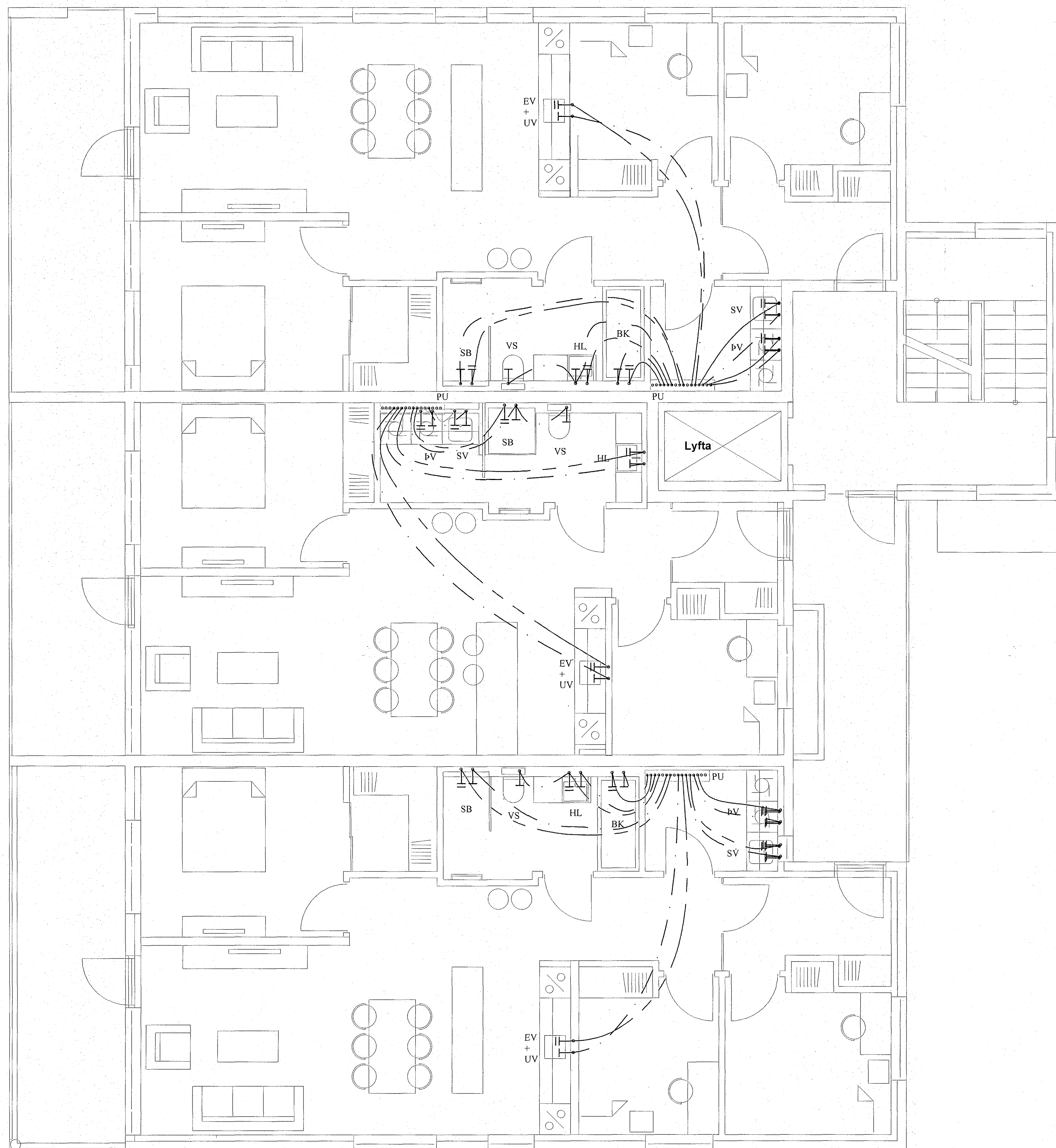
GRUNNMYND 2. HÆÐ MKV. 1:50
