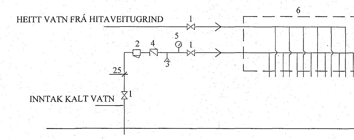
TENGRIND - NEYSLUVATN SKEMATÍSK
