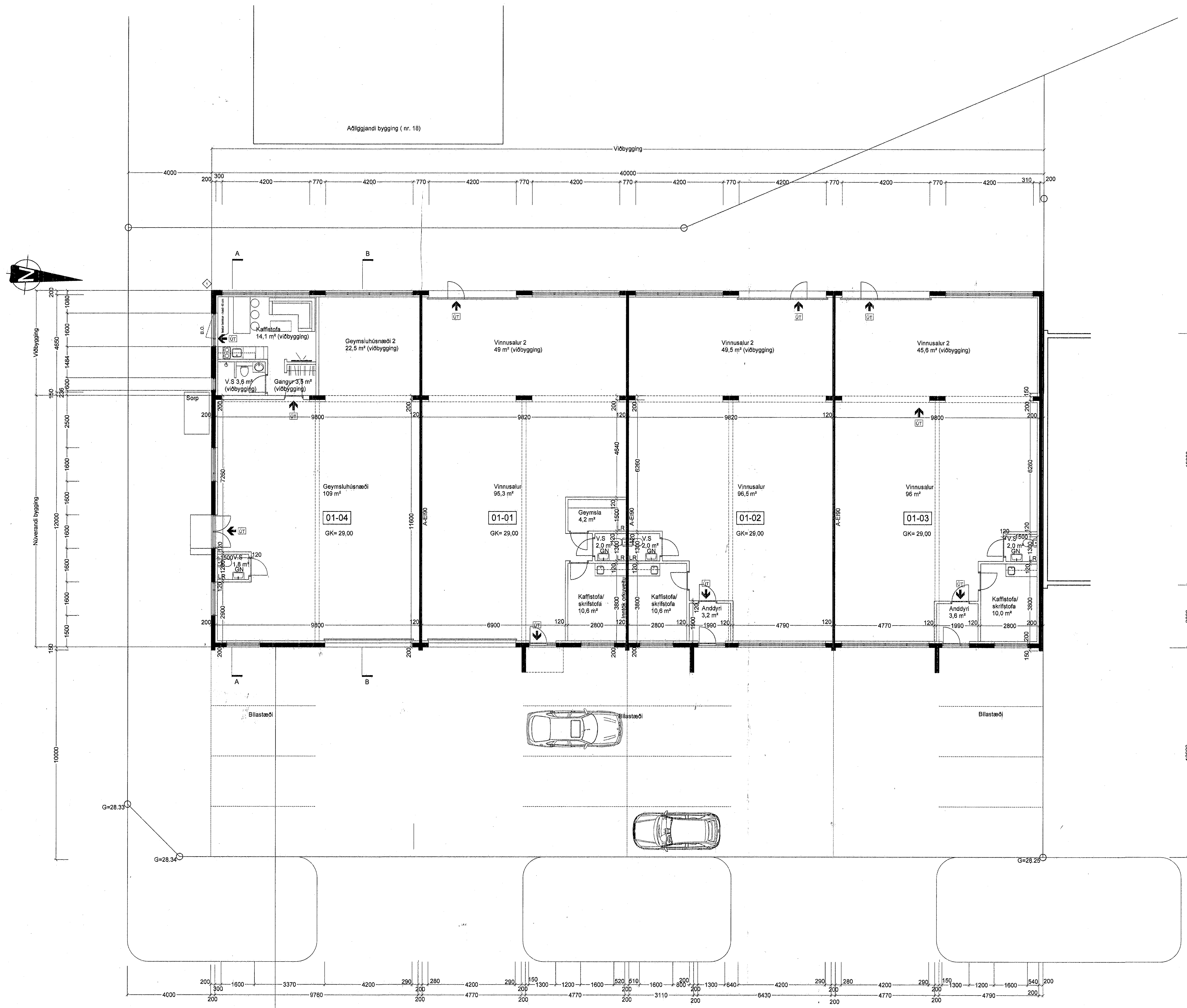
Grunnmynd 1. hæðar 1:100
