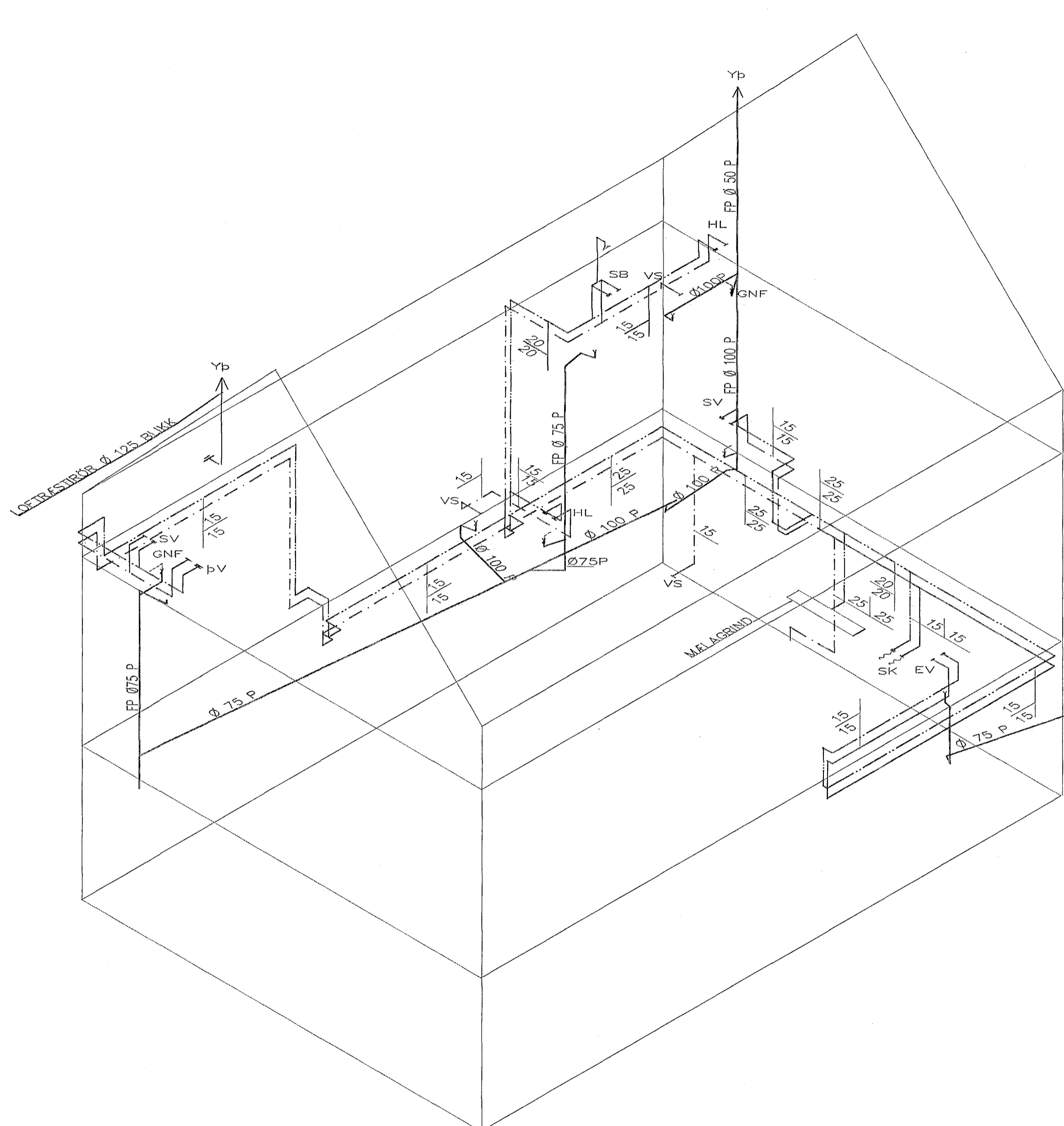
RÚMMYND VATNS OG FRÆRENNISLAGNA 1:50
