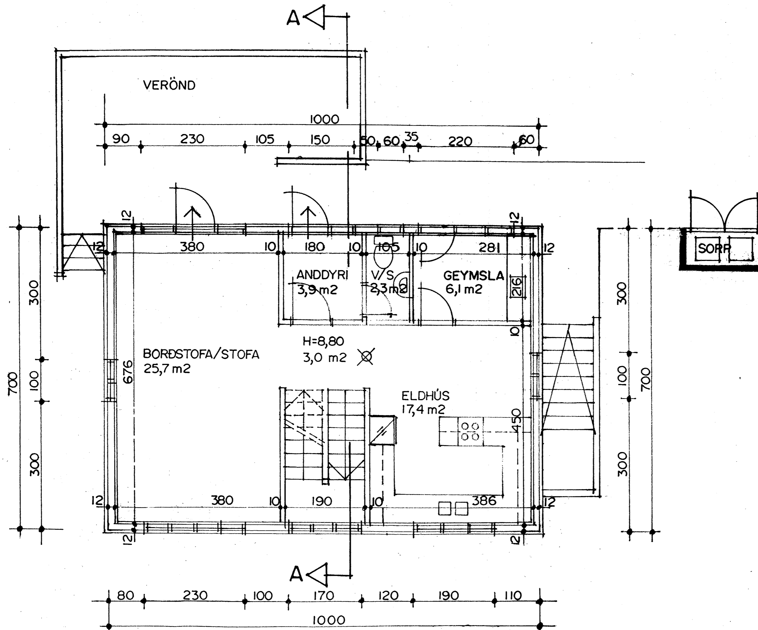
GRUNNMYND I HÆÐ MKV. 1:50.
