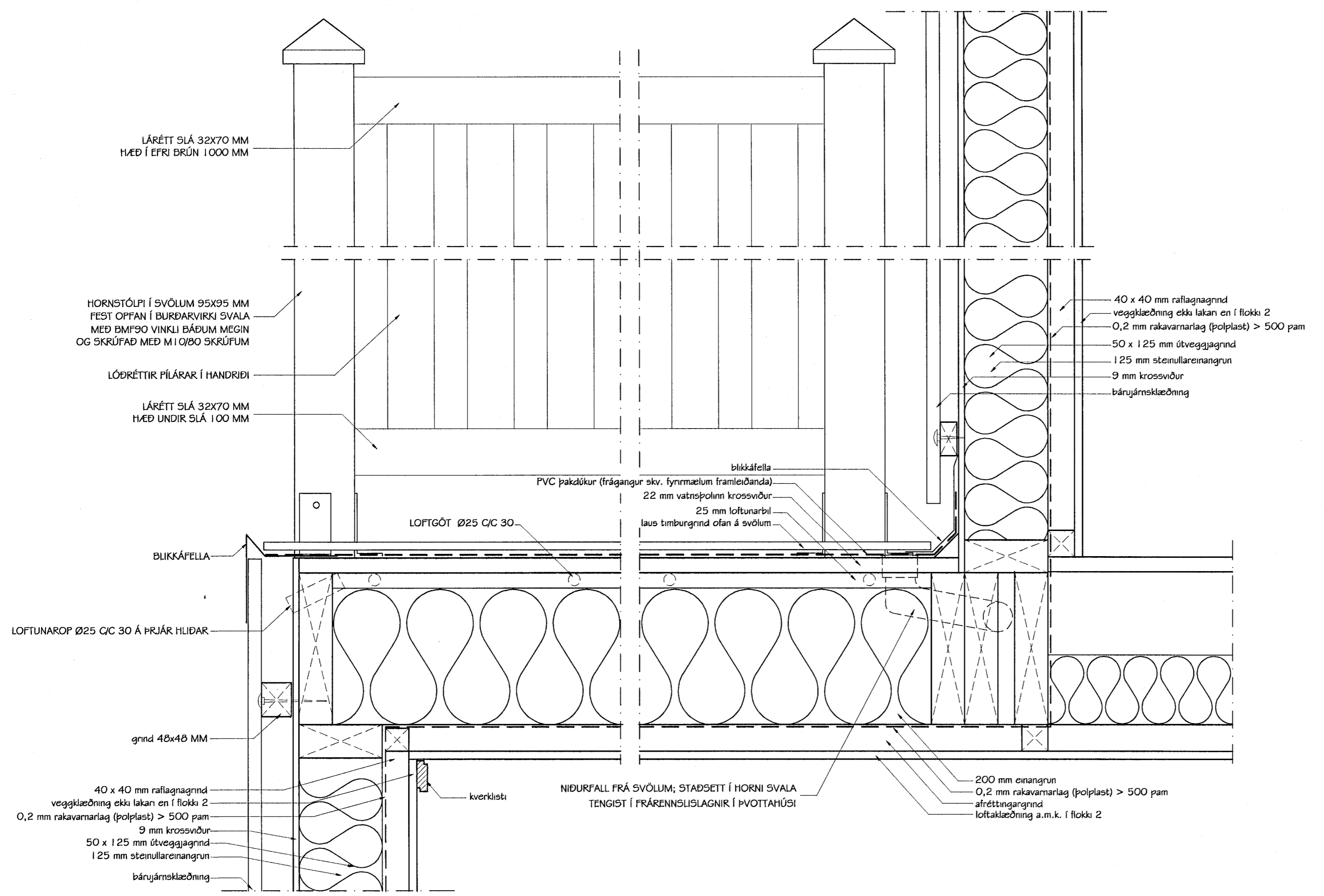
D9 FRÁGANGUR Á SVÖLUM MKV. 1:5
