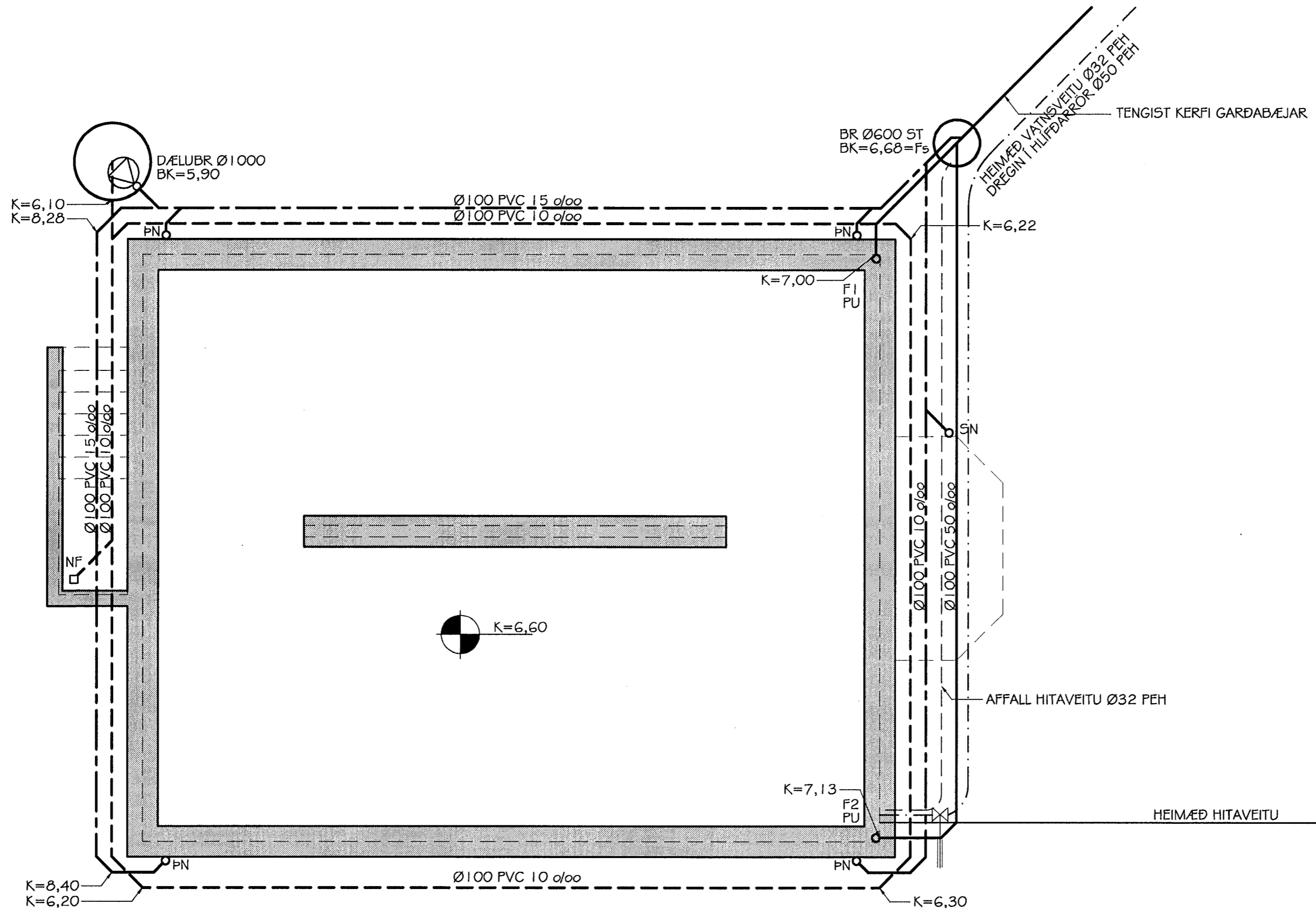
GRUNNMYND LAGNA Í JÖRD MKV. 1:50
