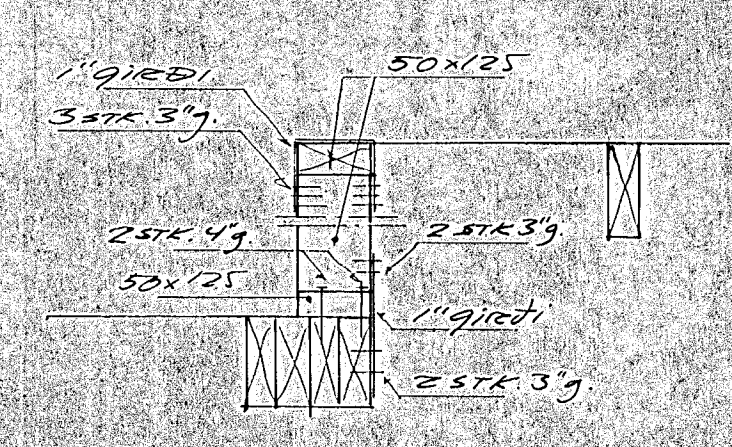
SNID L1-L1 1:20
