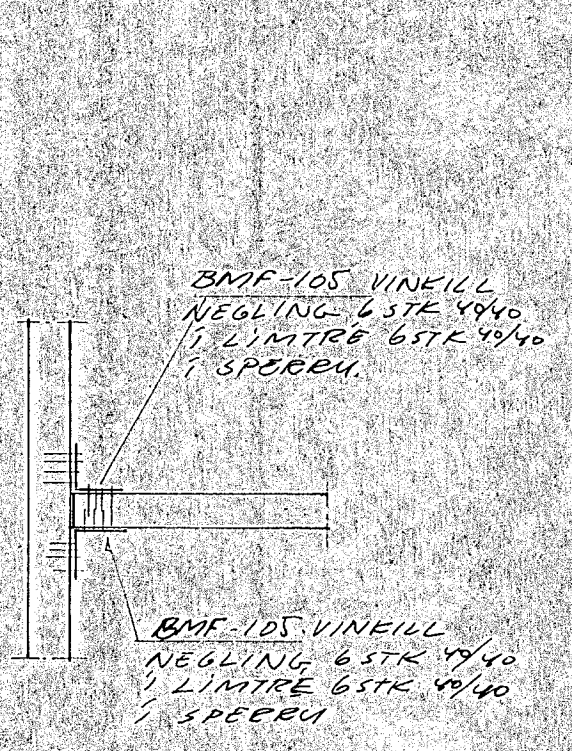
DEILI 2 1:10
