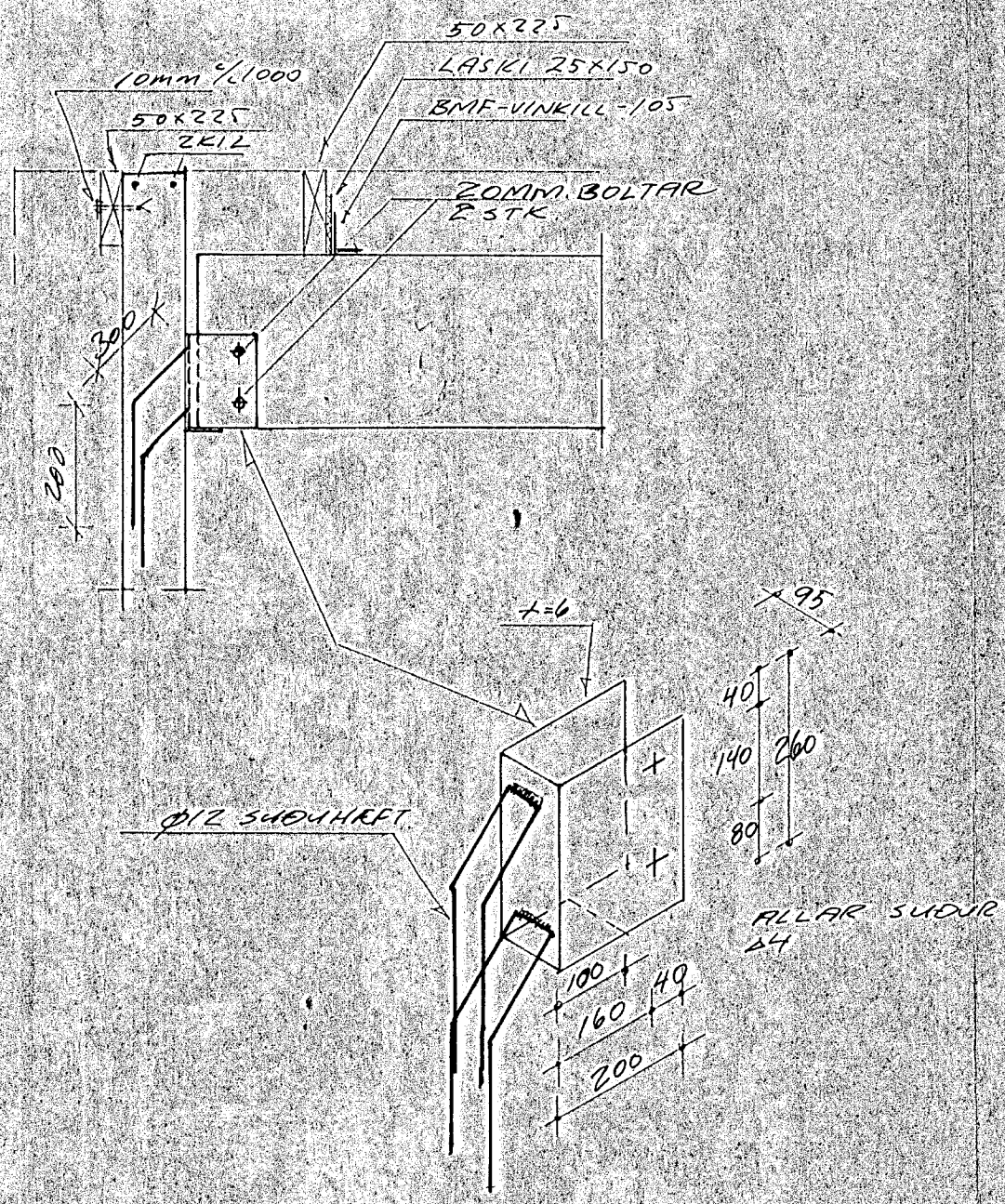
SNID A1-A1 1:20
