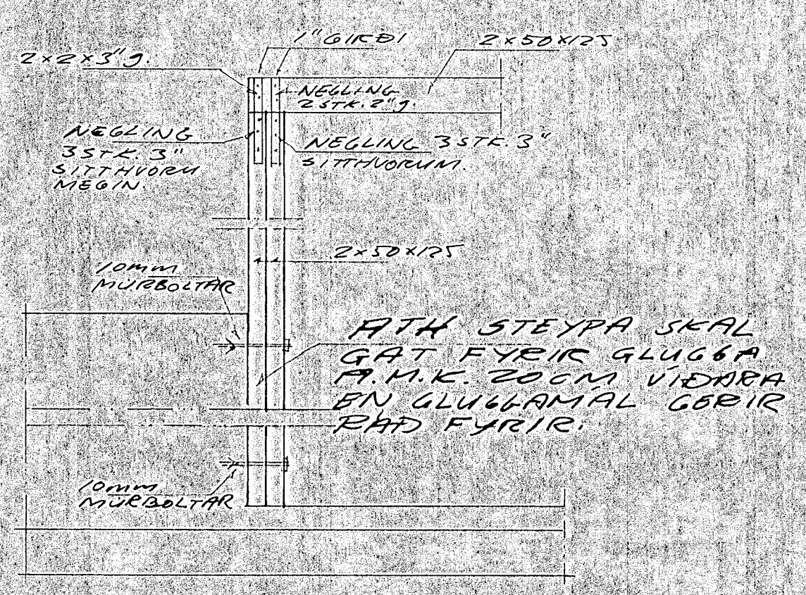
SNID M1-M1 1:20
