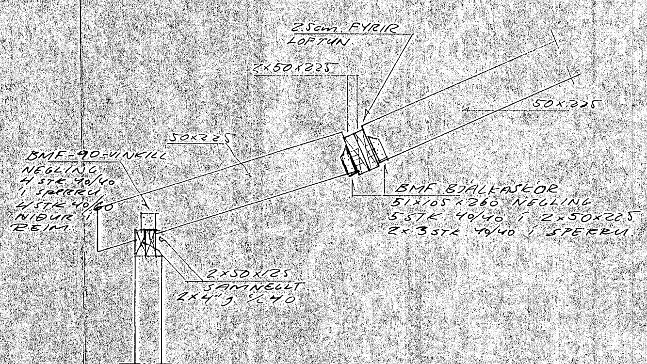
SNID M1-M1 1:20
