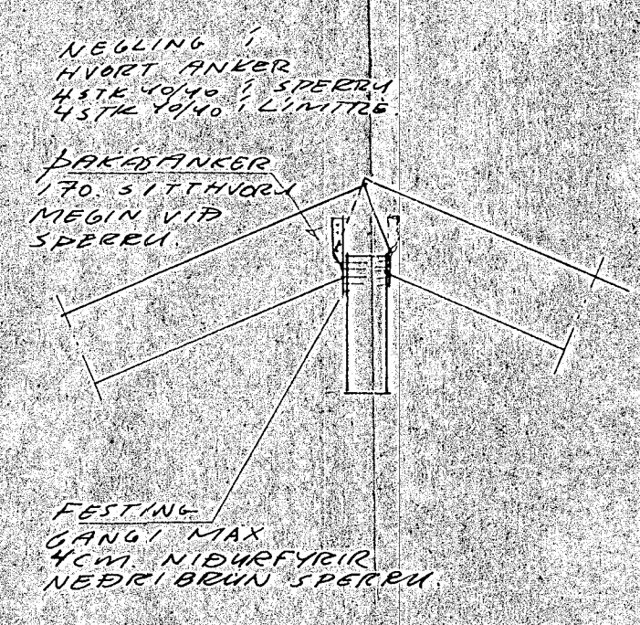
SNID I1-I1 1:20
