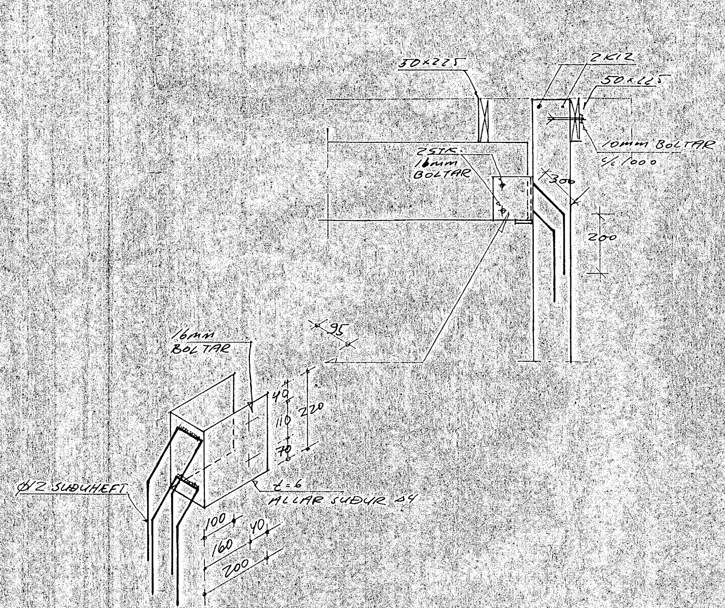
SNID F1-F1 1:20
