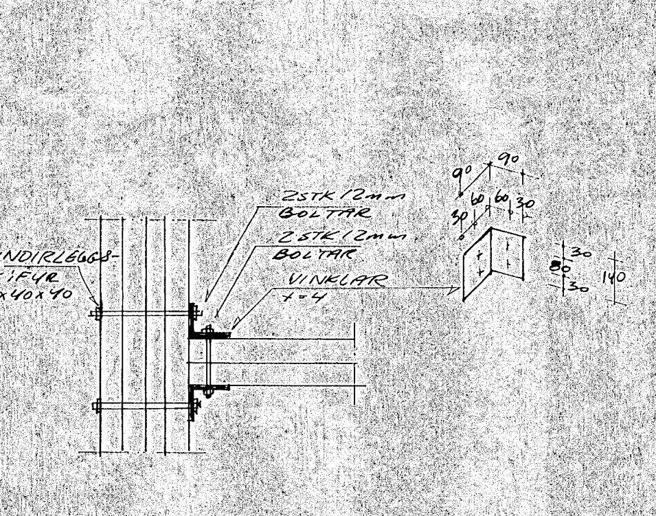
DEILI 3 1:10
