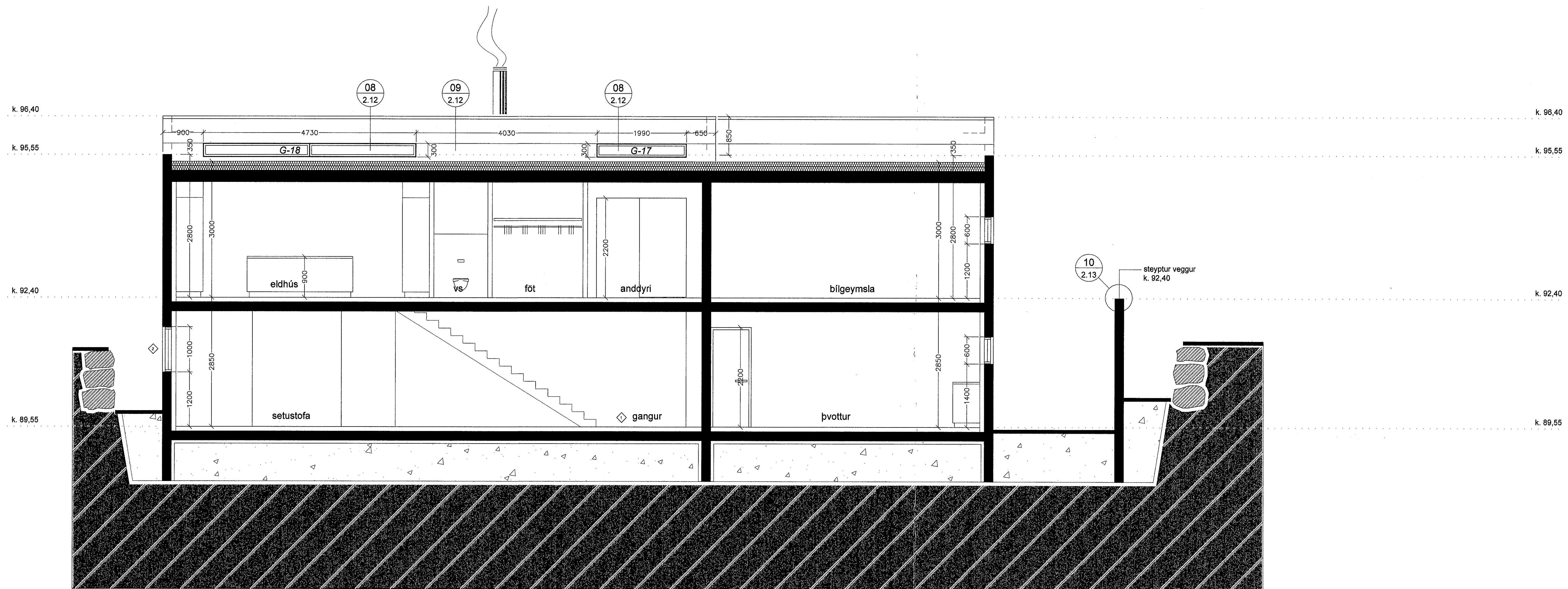
SNEIÐING E - E M 1 : 50
