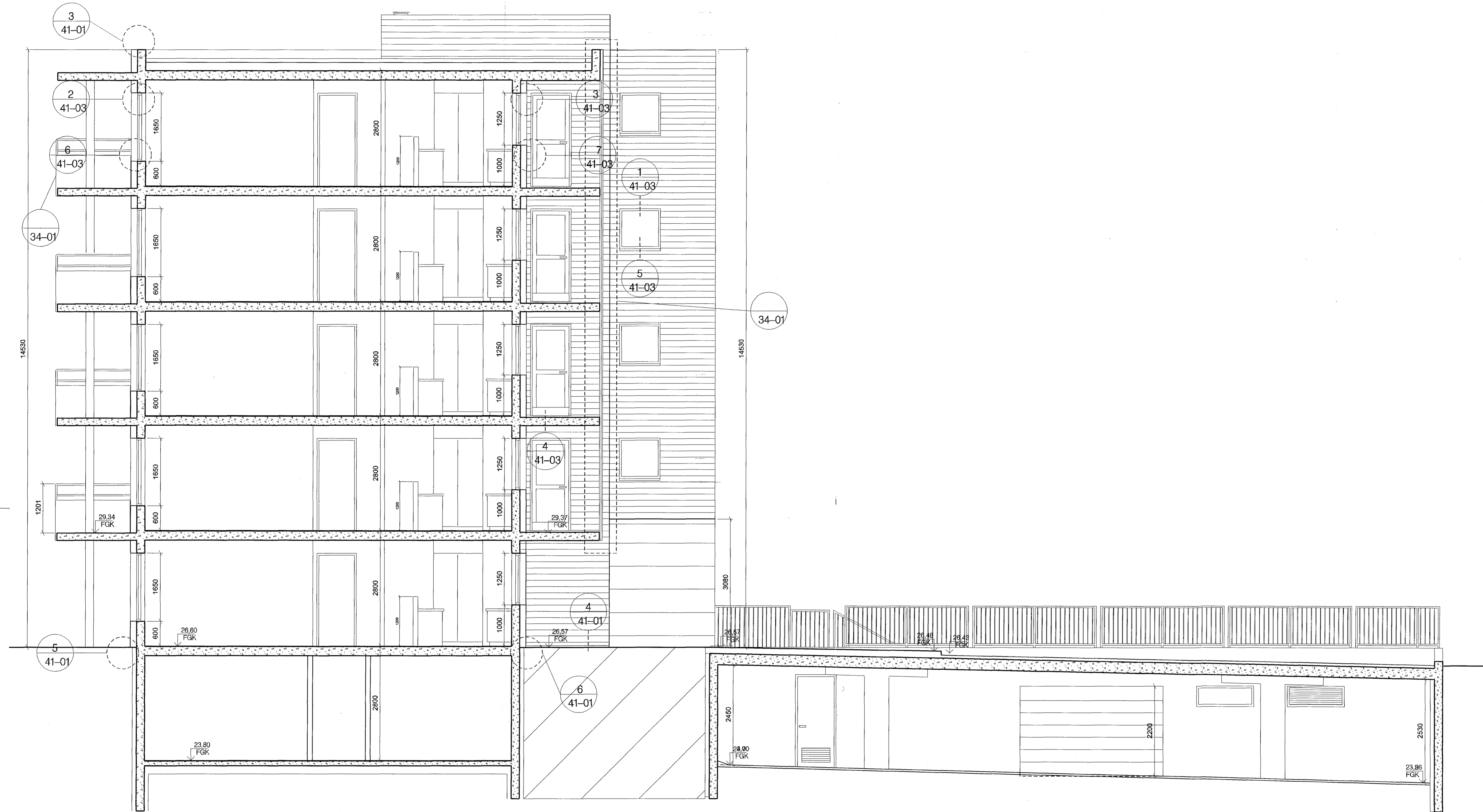
SNI* A-A 1:50
