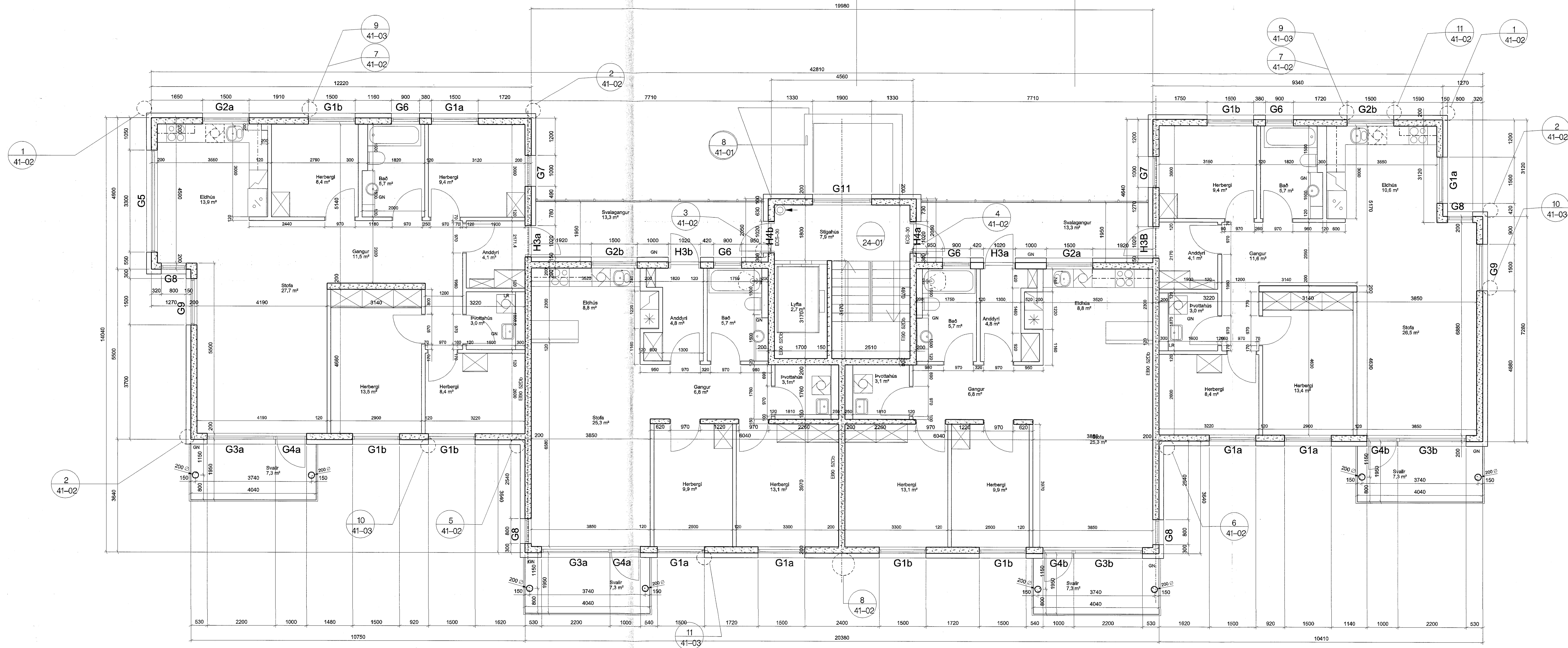
GRUNNMYND 1:50 2-5 hæð
