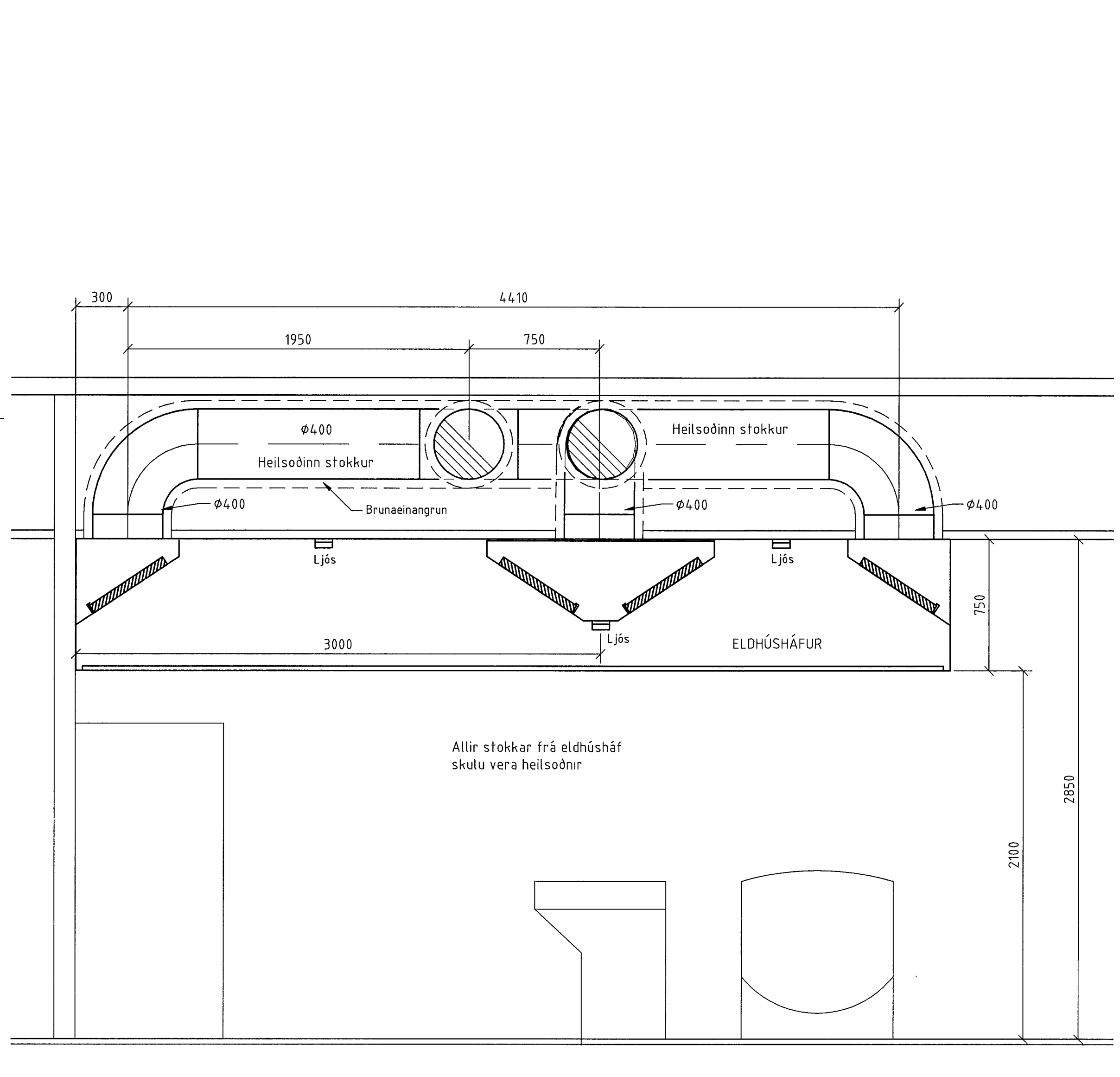
A 205/311 Snið Mkv. 1: 20
