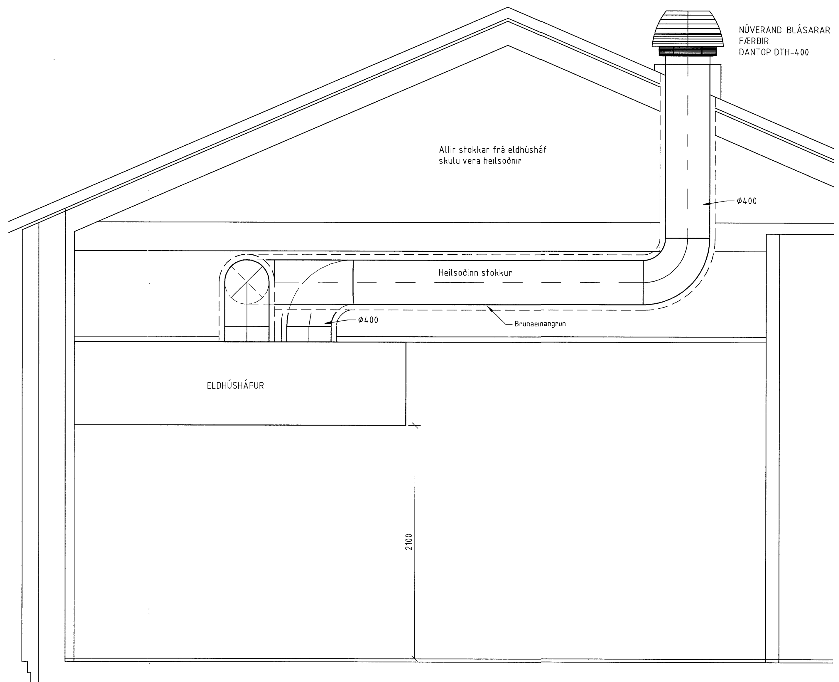
B 205/311 Snið Mkv. 1: 20
