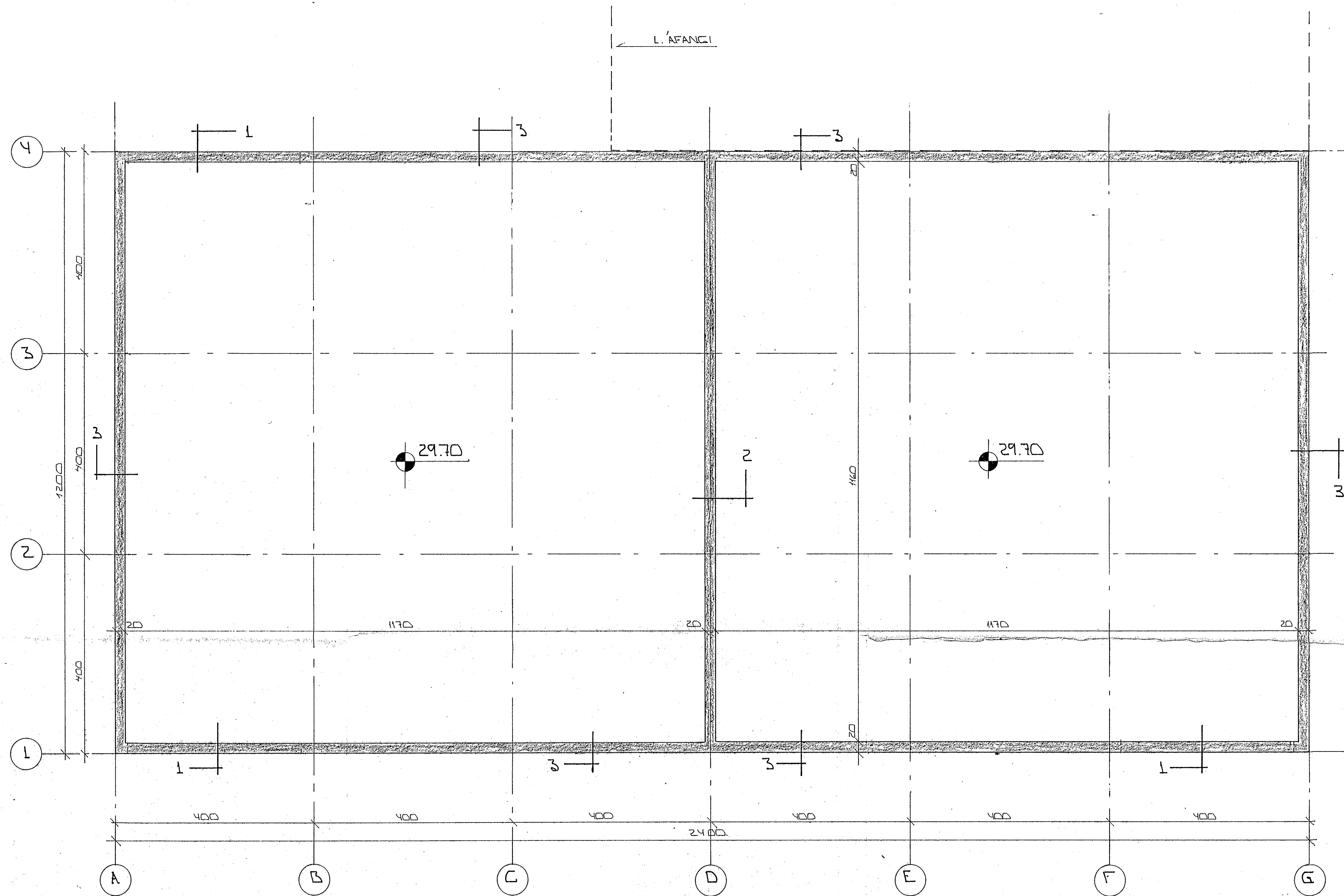
GRUNNMYND 1:50
