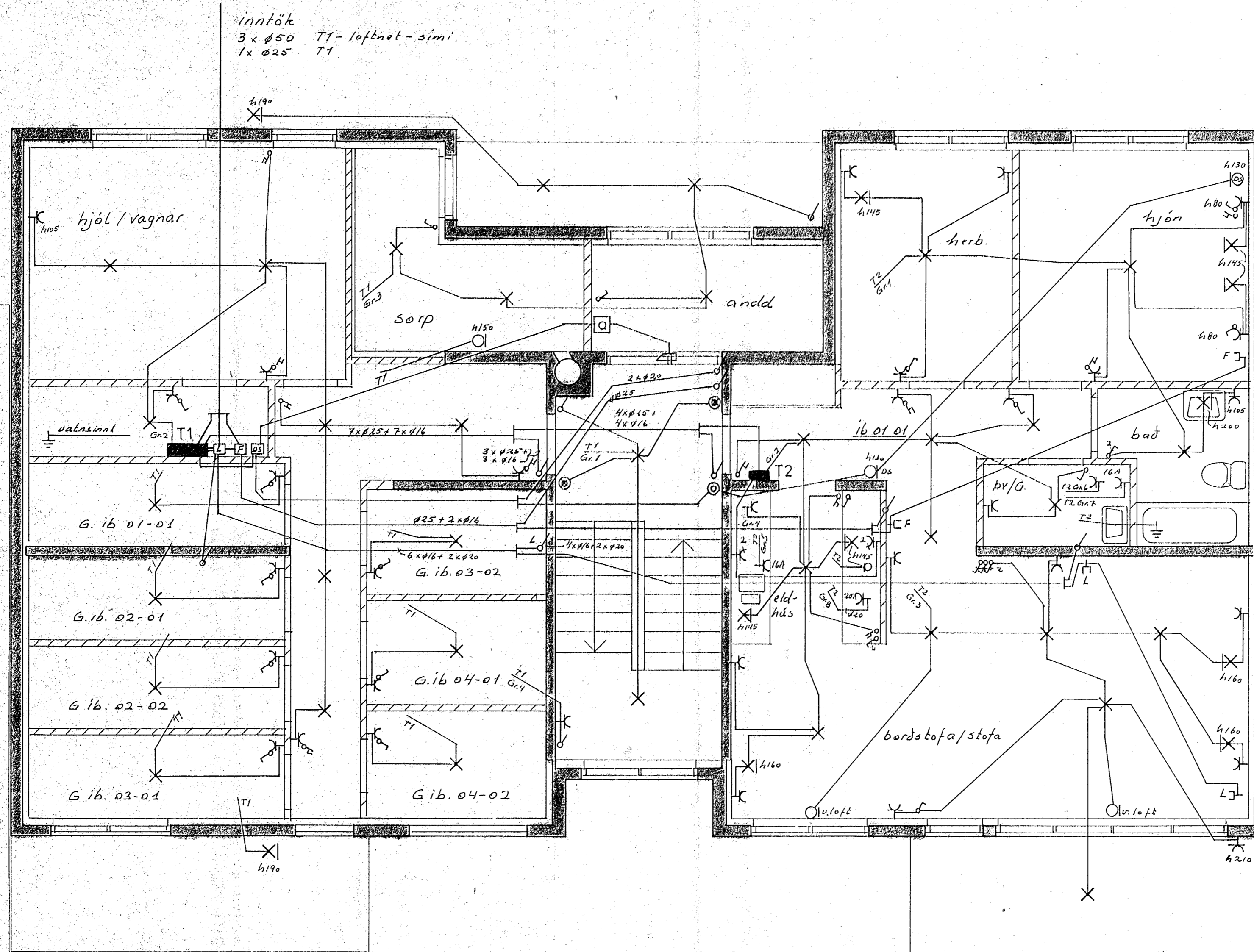
GRUNNMYND 1 HÆÐAR M. 1:50
