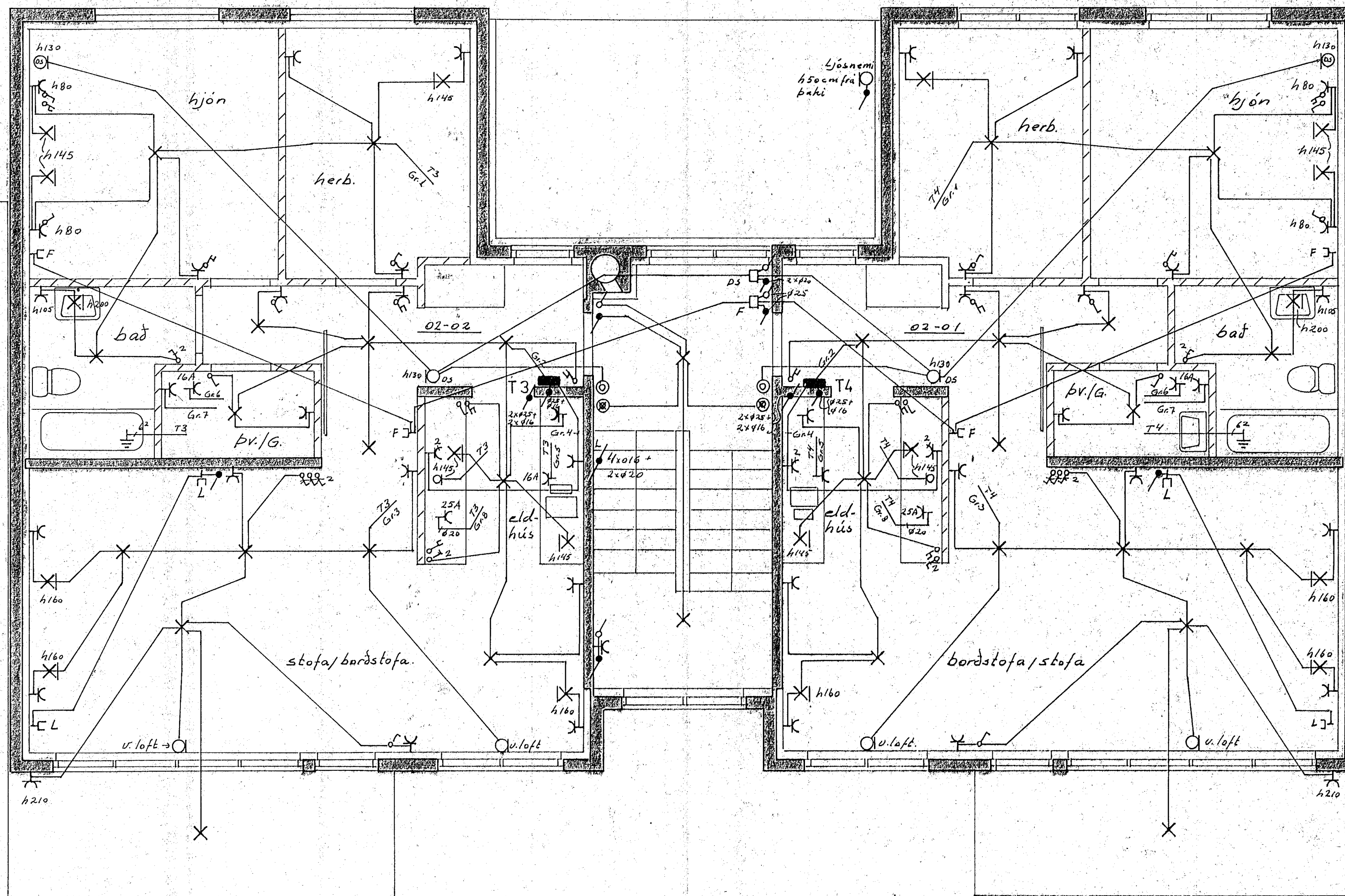
GRUNNMYND 2. HÆÐAR M. 1:50
