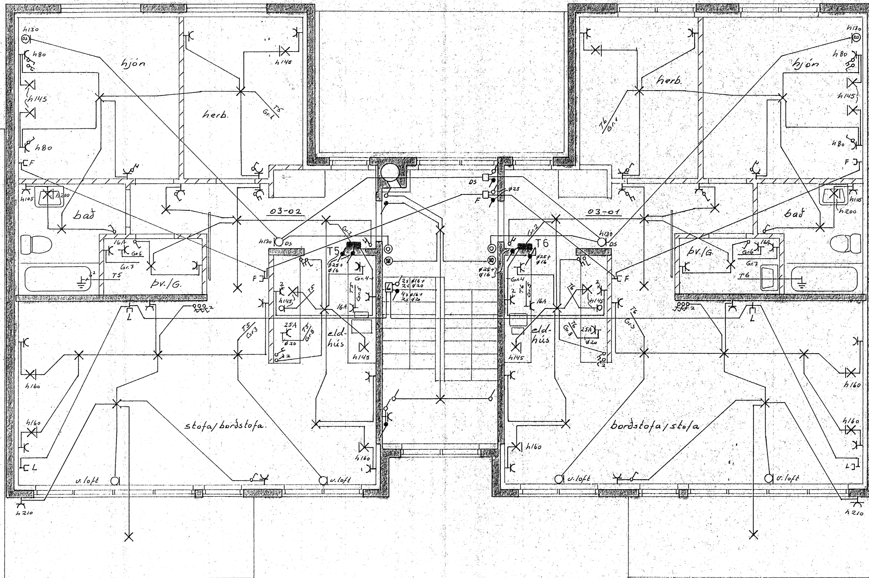
GRUNNMYND 3. HÆÐAR M. 1:50
