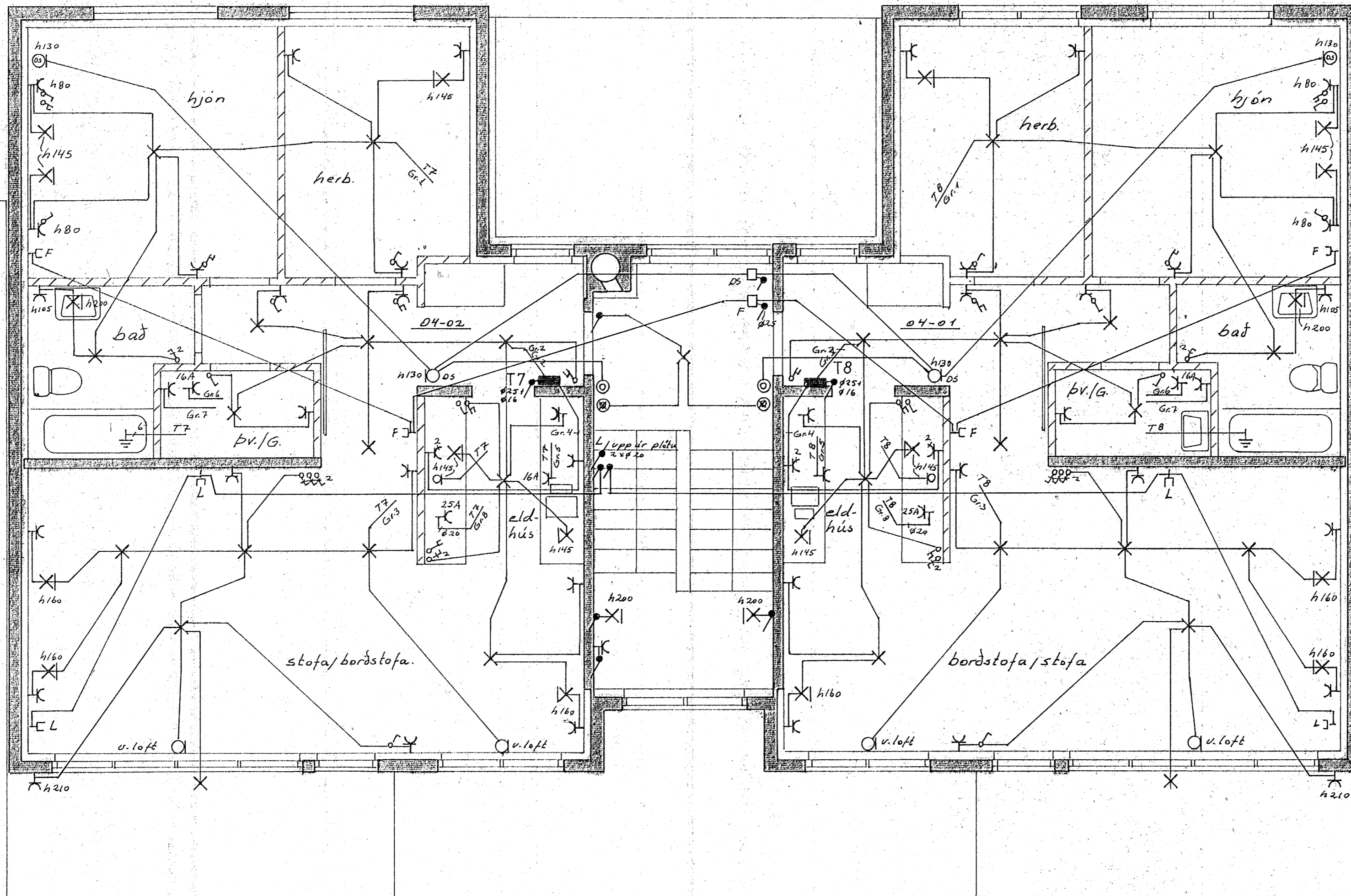
GRUNNMYND 4. HÆÐAR M. 1:50
