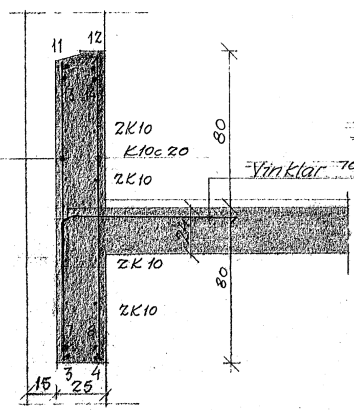
B-B 1:20.
