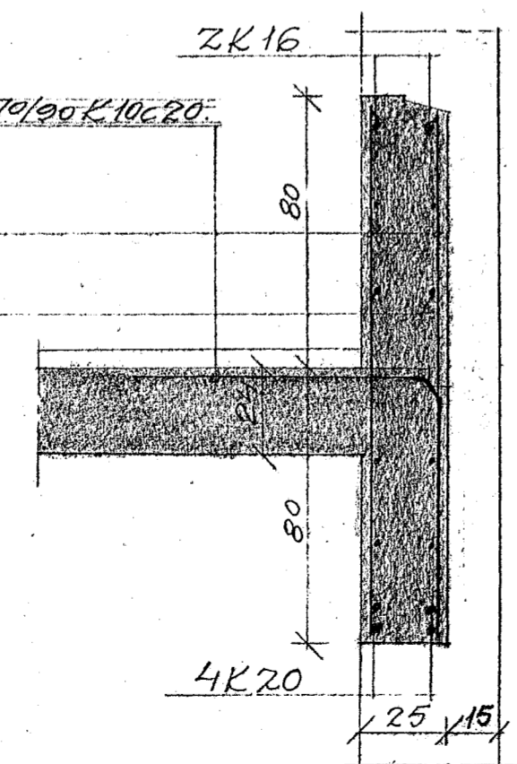
D-D 1:20.
