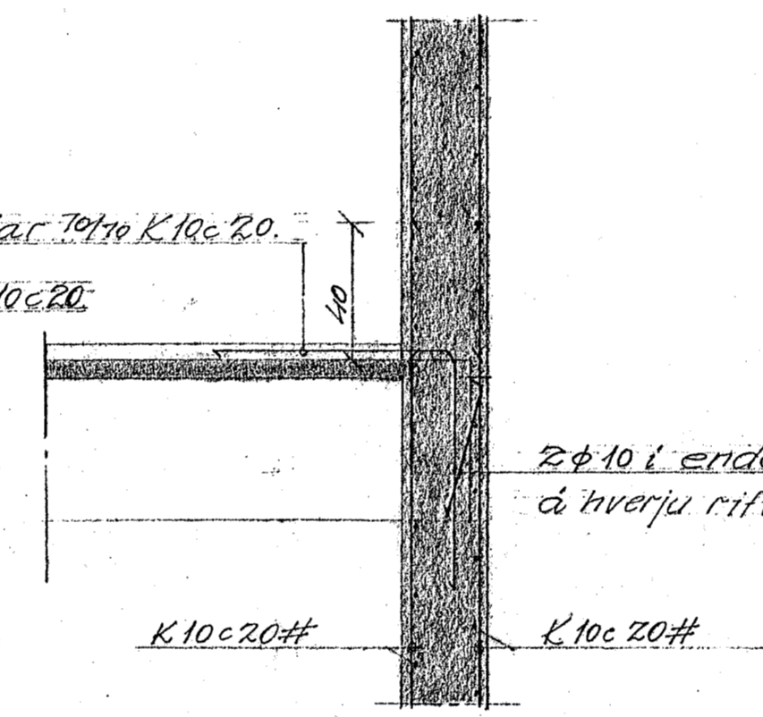
E-E 1:20.
