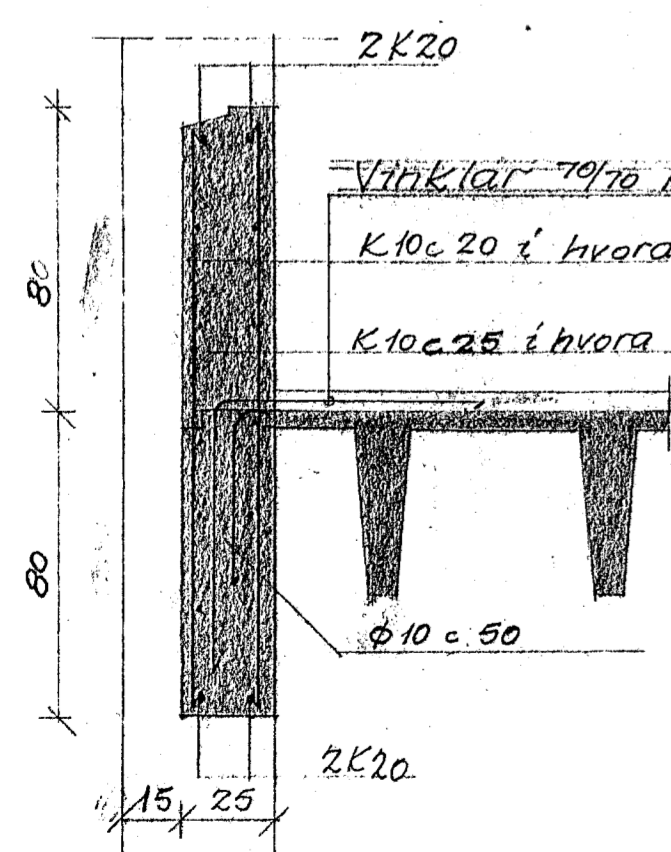
C-C 1:20.
