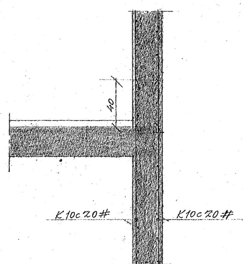
F-F 1:20.
