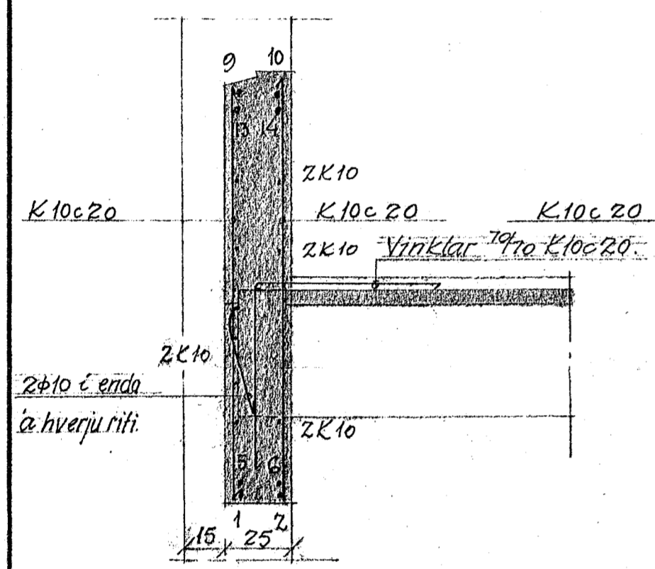
A-A 1:20.
