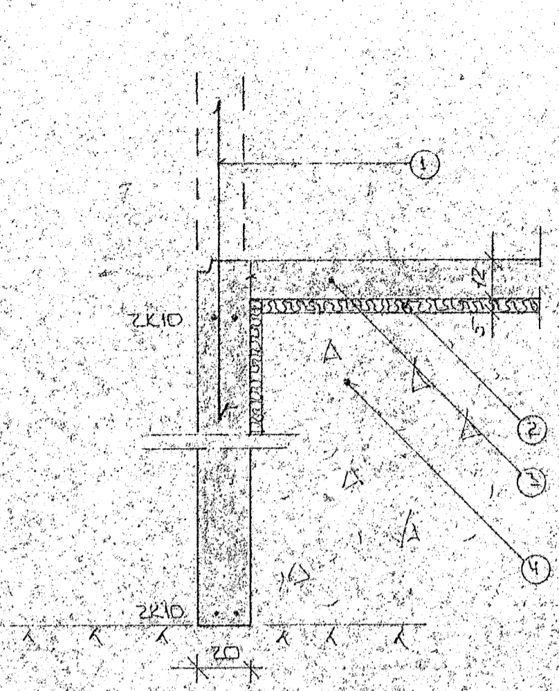
SNID 1 Í UTVEGGI 1:20
