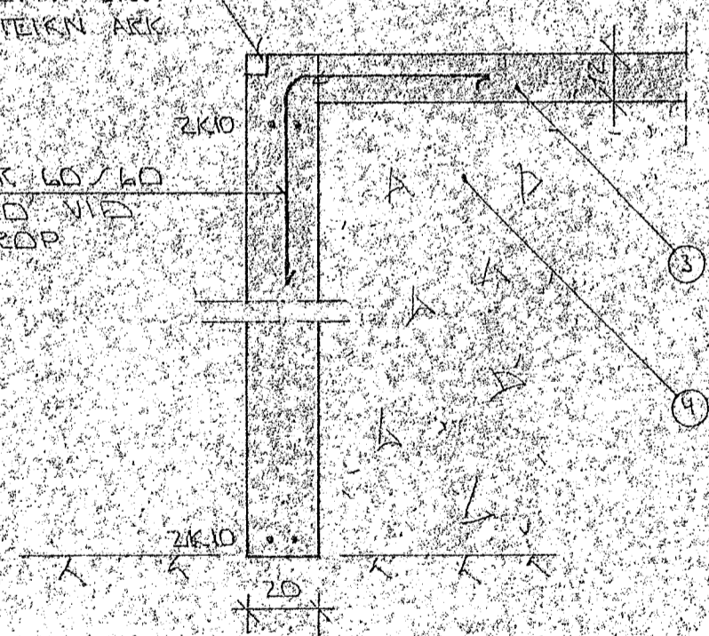
SNID 2 Í HURDAROP Á BÍLG. 1:20
