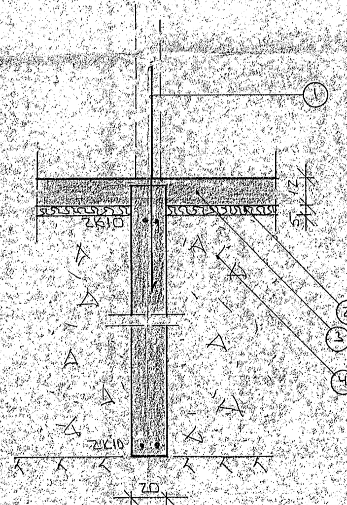
SNID 4 Í MILLIVEGG 1:20
