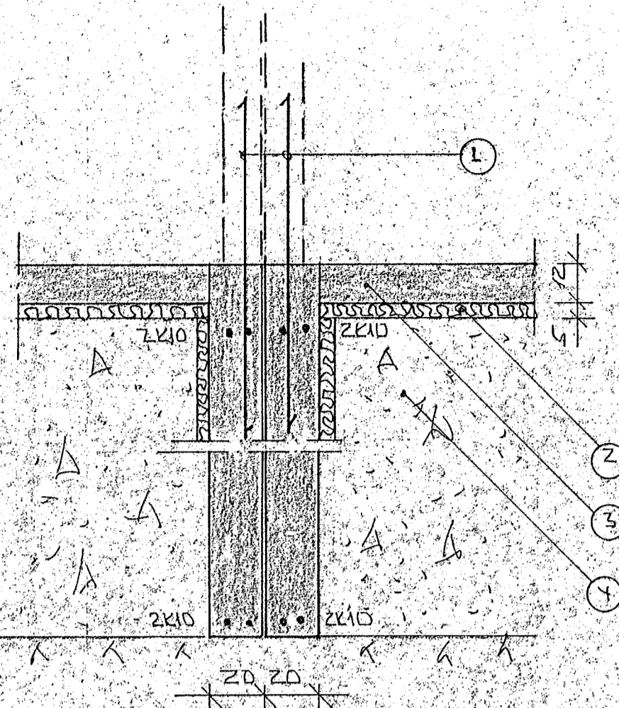
SNID 3 MILLI HUSA 1:20
