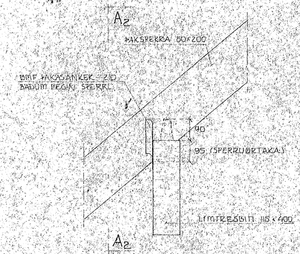
SNID A2-A2 m.kv. 1:10
