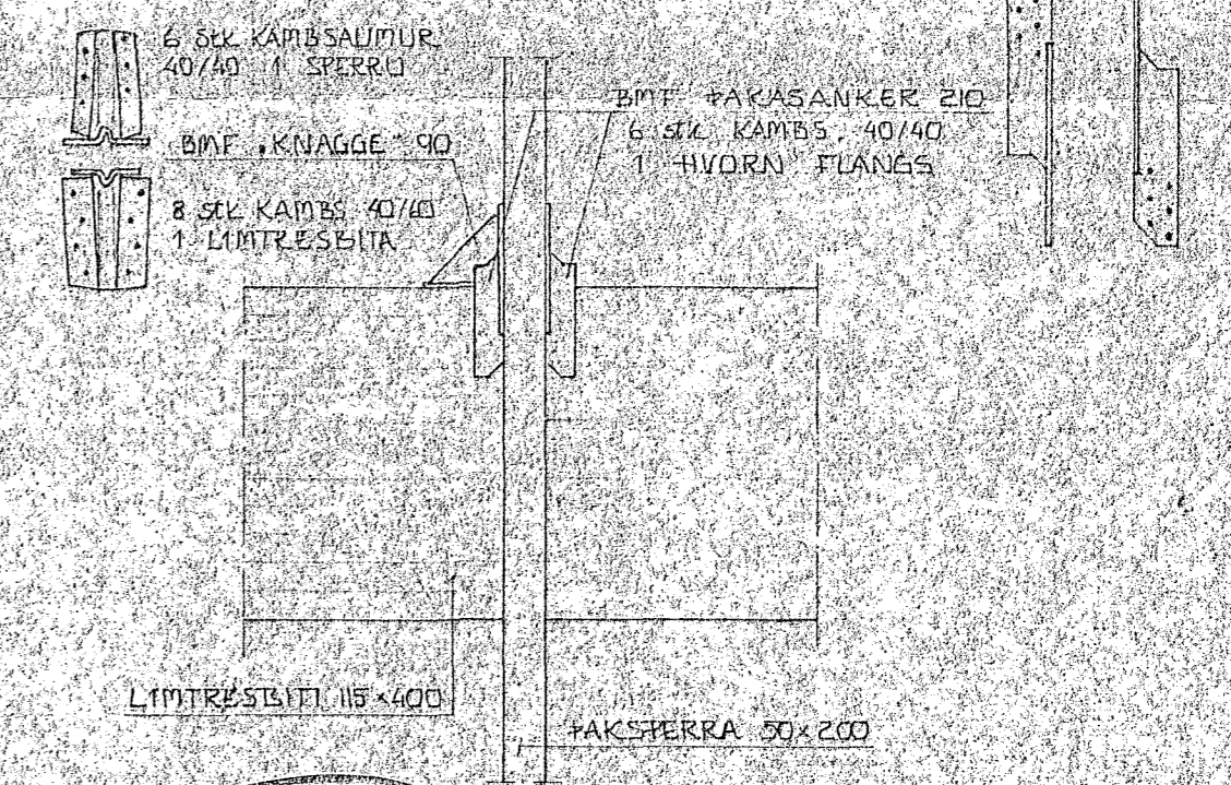
SNID A2-A2 m.kv. 1:10
