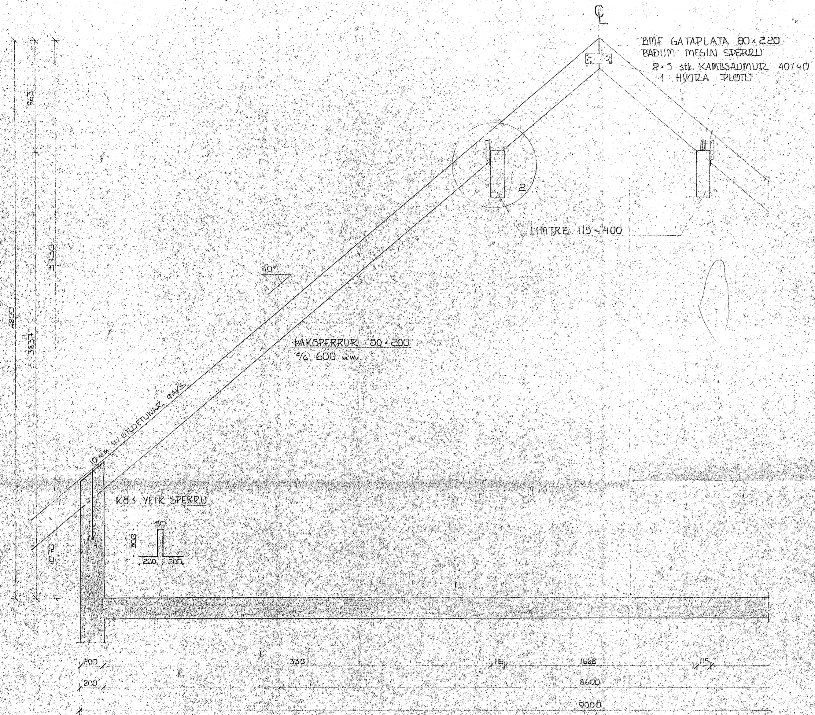
SNID A-A m.kv. 1:20
