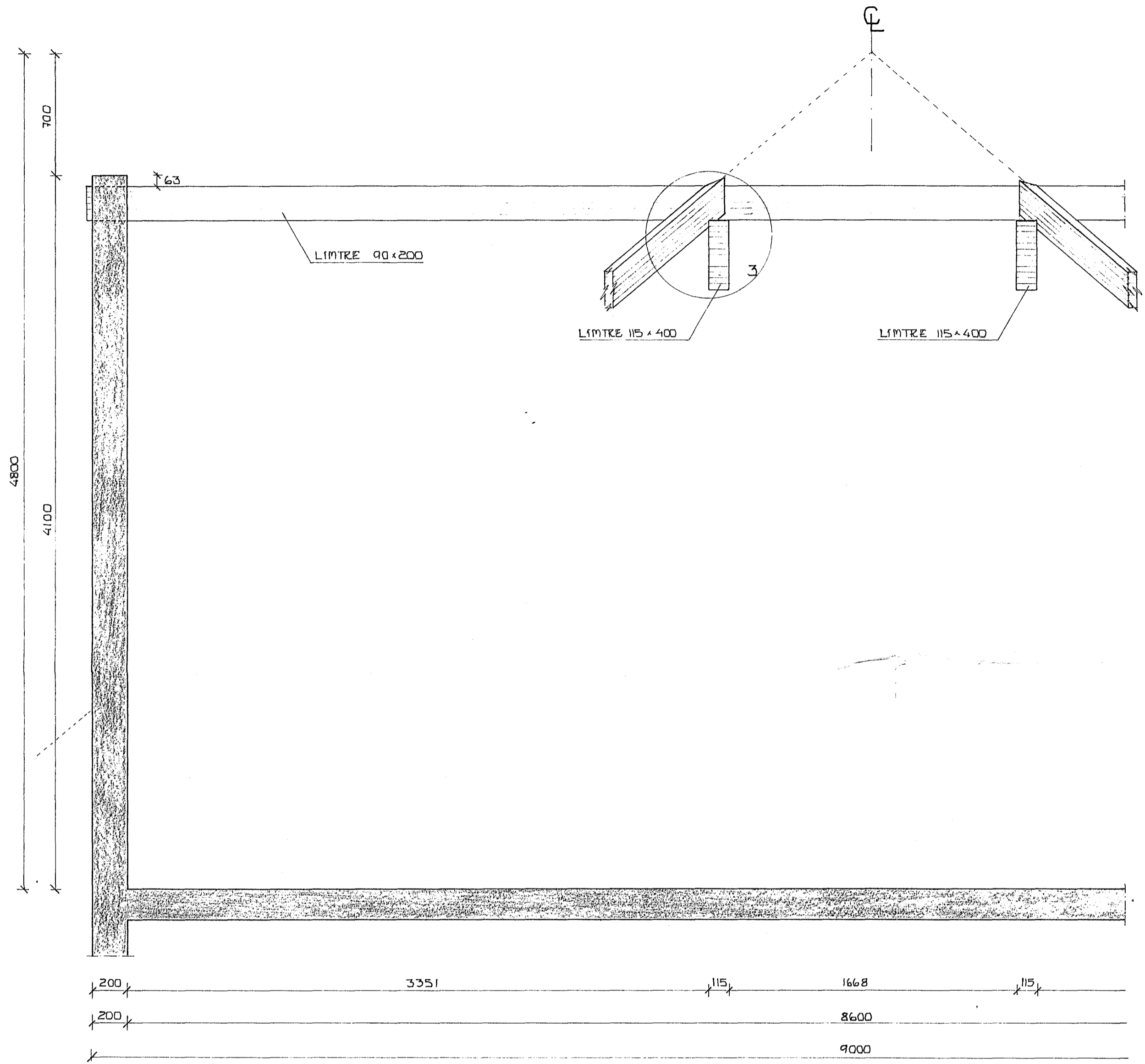
SNID B-B. Mkw. 1:20.
