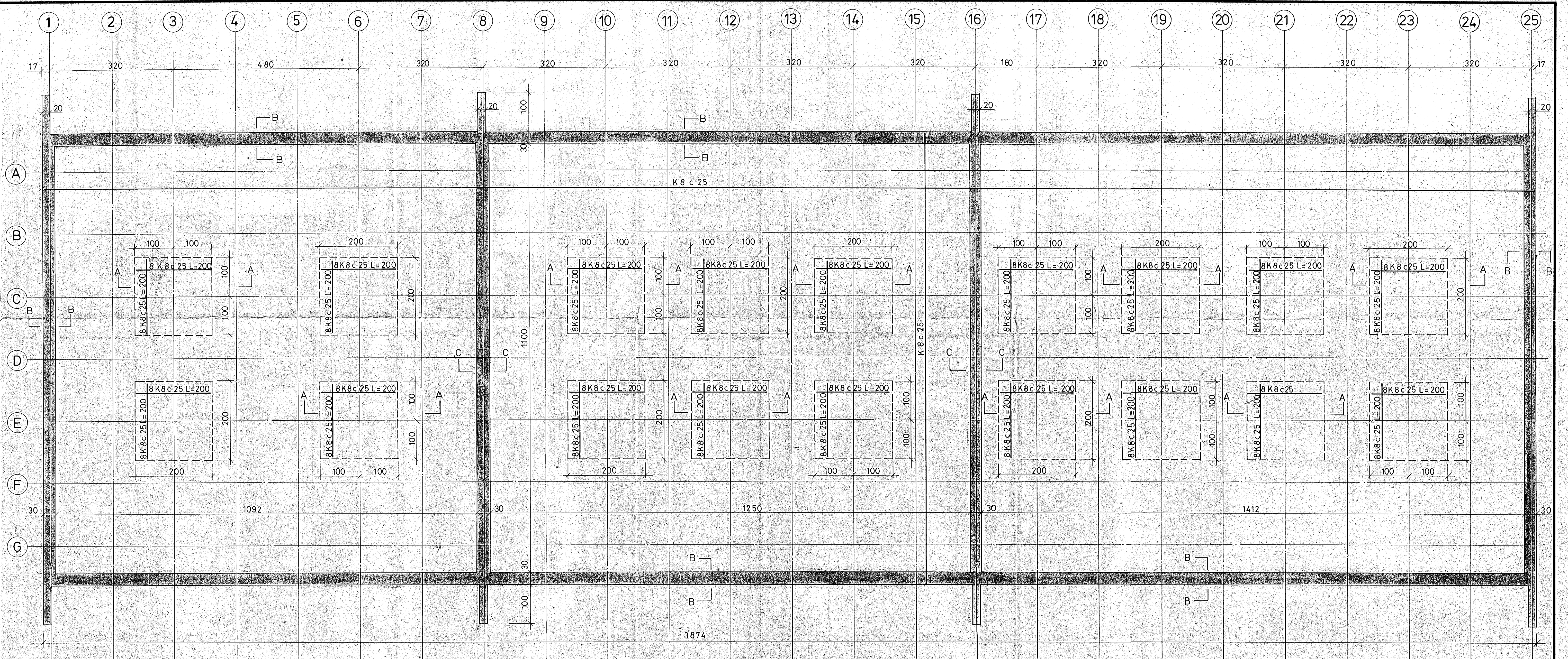
GRUNNMYND 1:50
