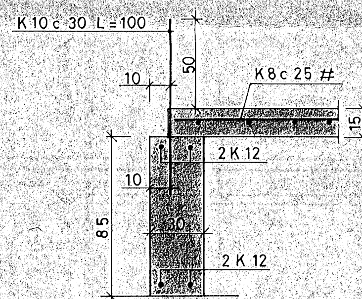
SNID B-B 1:20
