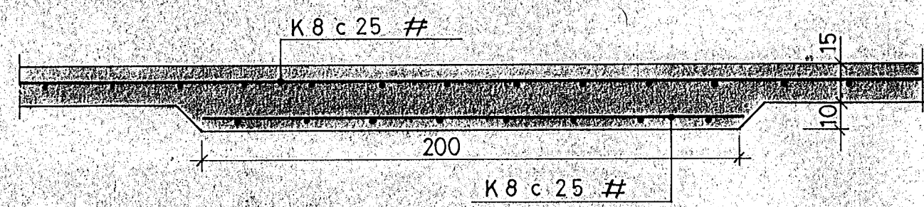
SNID A-A 1:20
