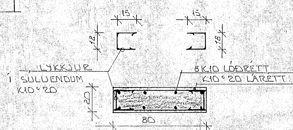
SNID Í SÚLU S1 1:20 (ÚTVEGGJUM) 1-03
