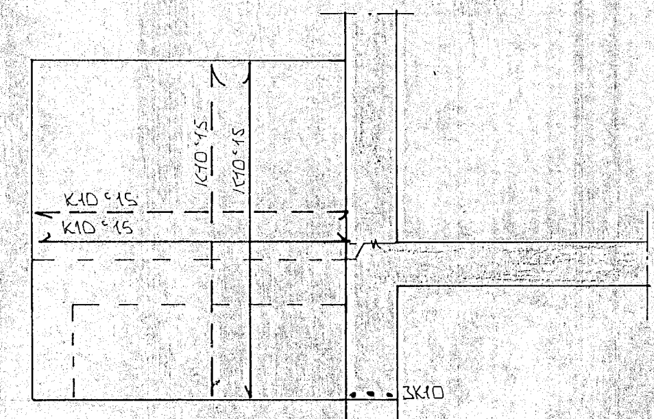
BENDING VEGGJA Í SVÖLUM 1:20
