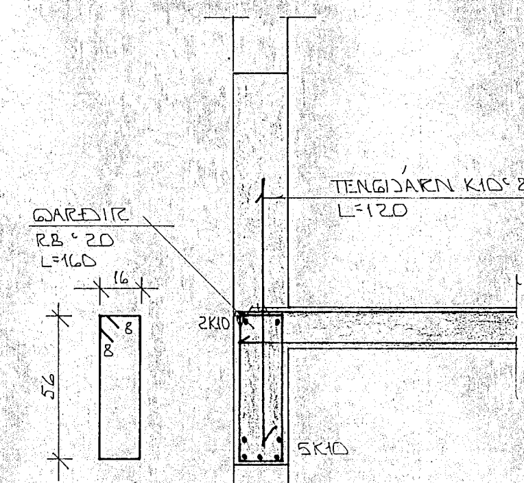
SNID Í BITA YFIR GLUGGUM 1:20
