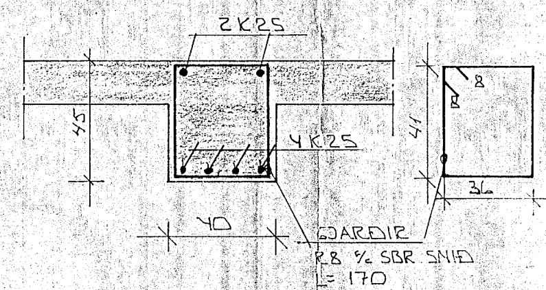
SNID 7-7 Í BITA 1:20 1-03
