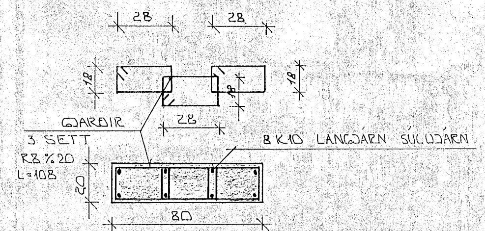
SNID Í SÚLU S2 1:20 (INNVEGGJUM) 1-03
