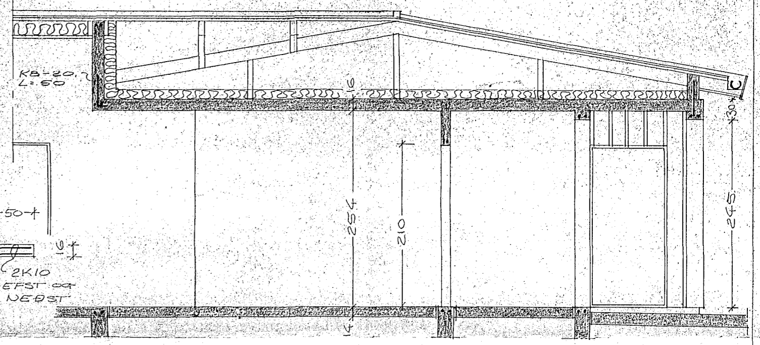
SKURÐUR A-A, M=1:50
