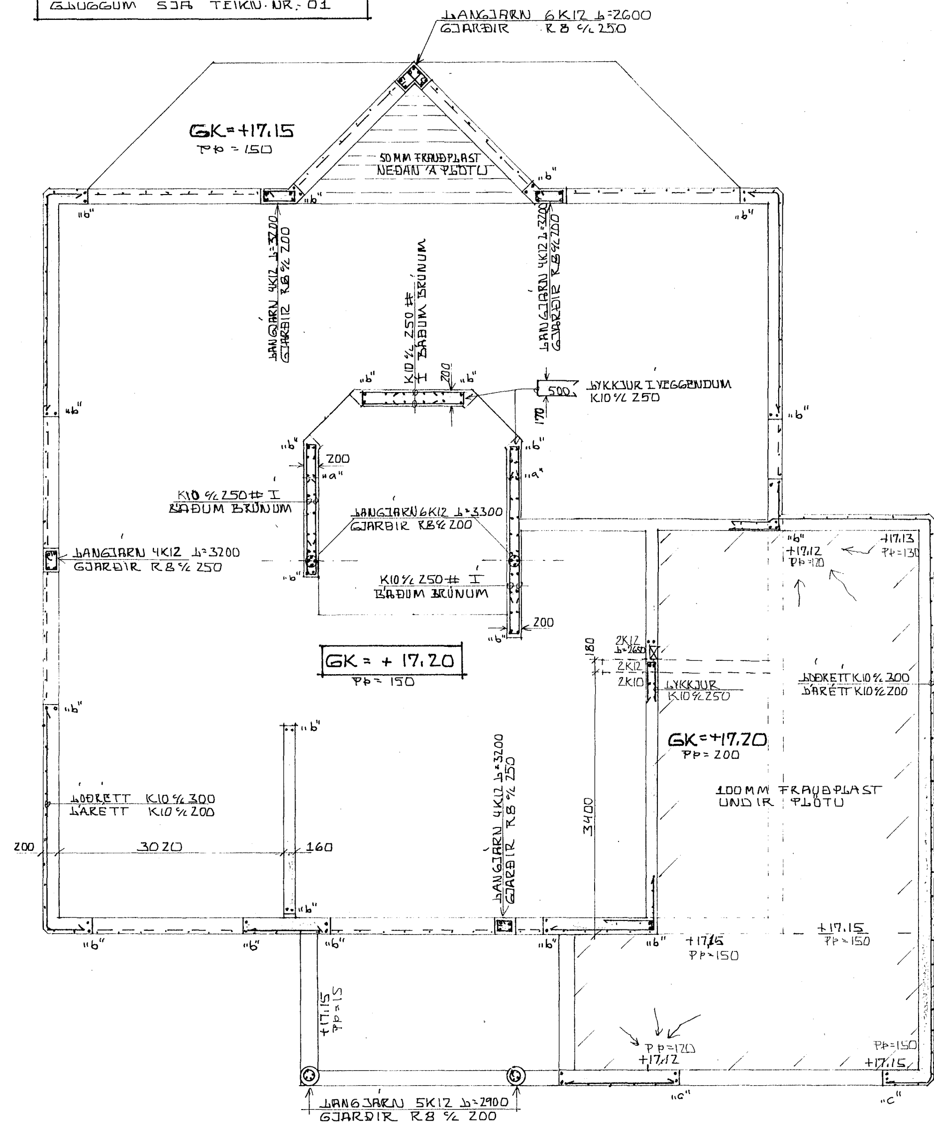
GRUNMYND 1:50
