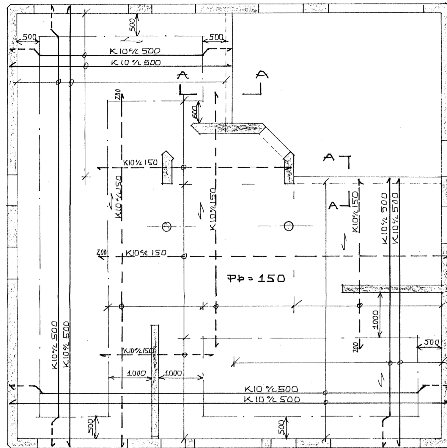
GRUNNMYND 1:50
