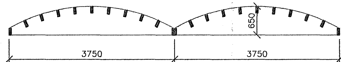
ÞVERSIND Í SPERRUPLAN MKV. 1:50
