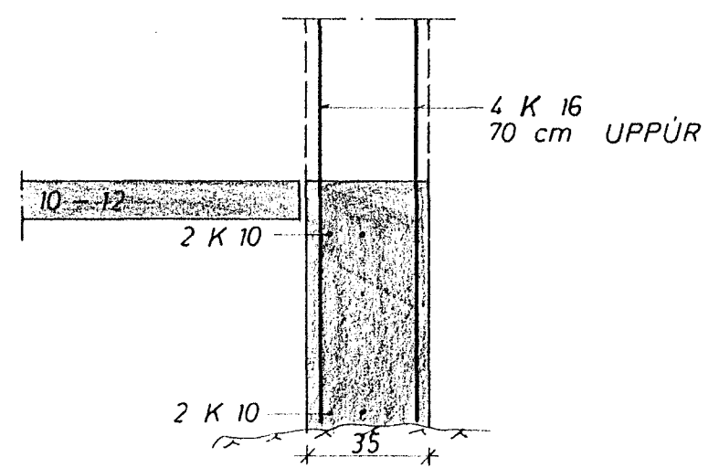
SNIÐ B 1: 20 SÜLUUNDIRSTÖÐUR
