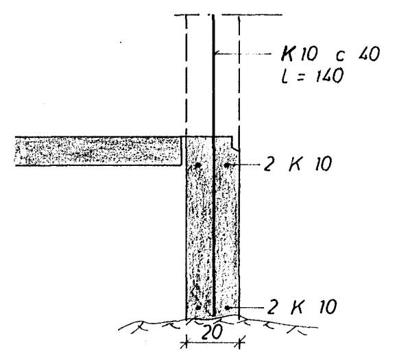
SNIÐ A 1: 20
