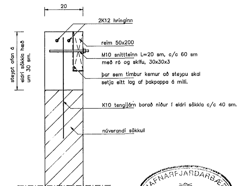
Snið Y-Y Mkv. 1 : 50
