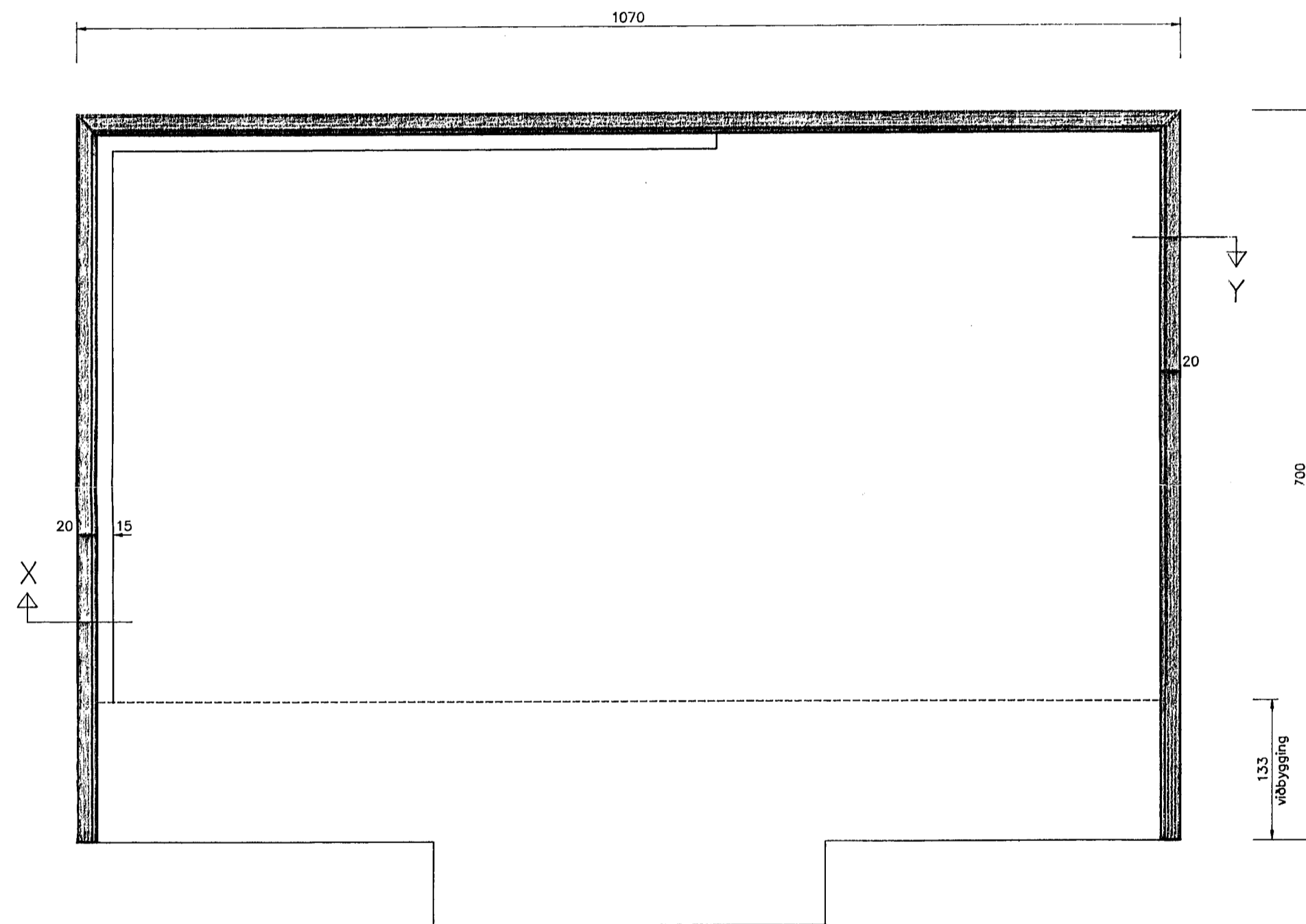
Styrking á sökklum Mkv. 1 : 50
