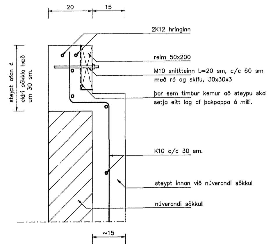
Snið X-X Mkv. 1 : 50
