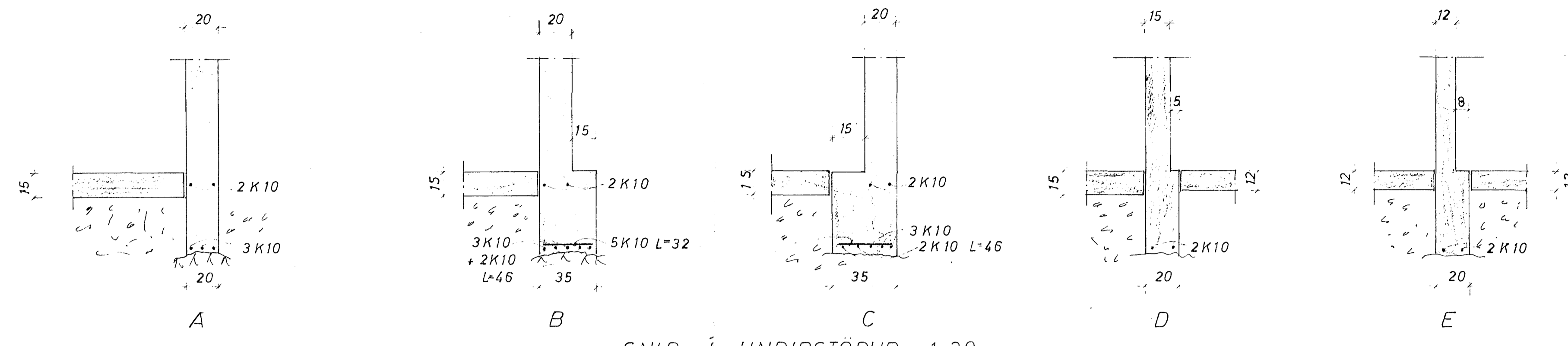
SNID Í UNDIRSTÖÐUR 1:20
