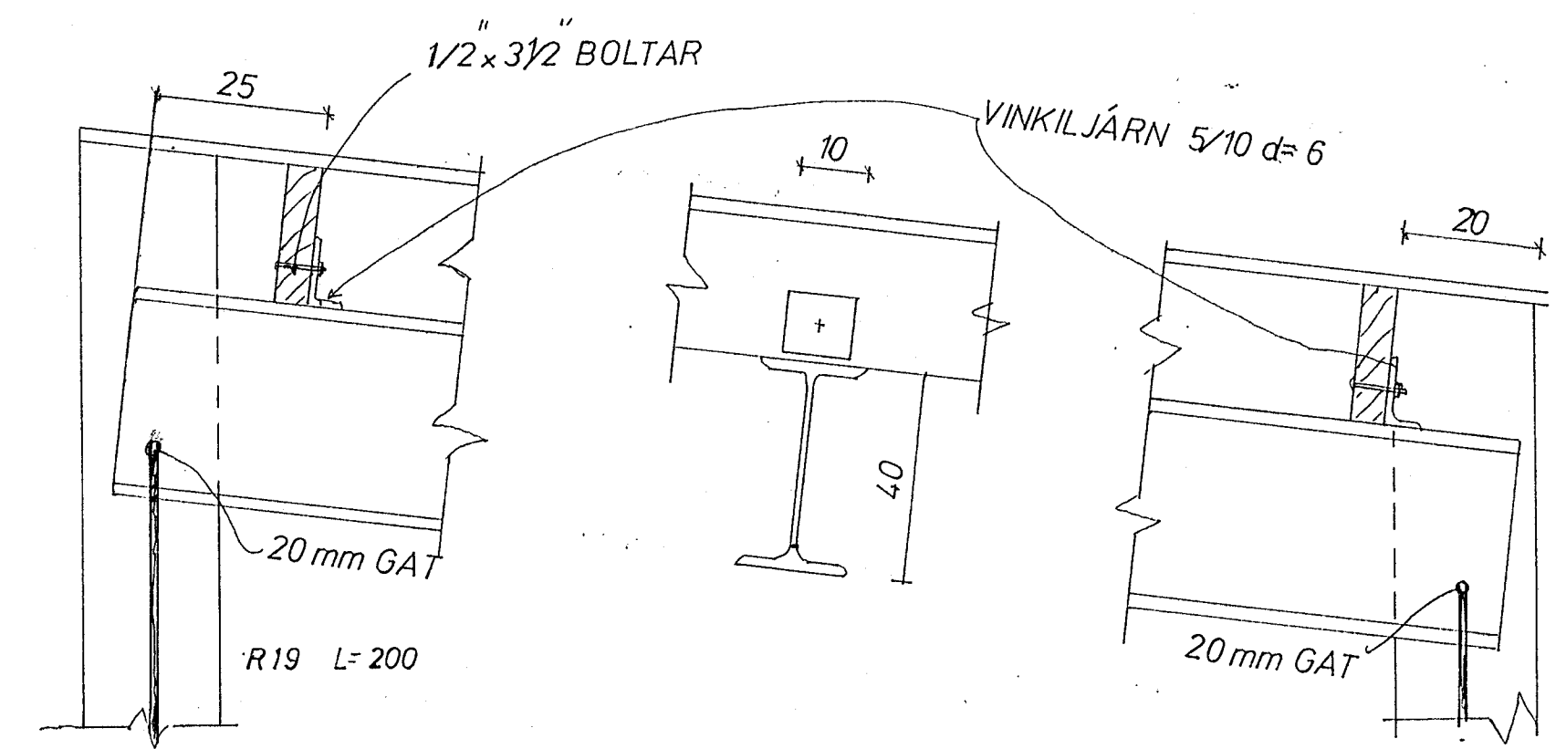
BITA OG SPERRUFESTINGAR 1:10
