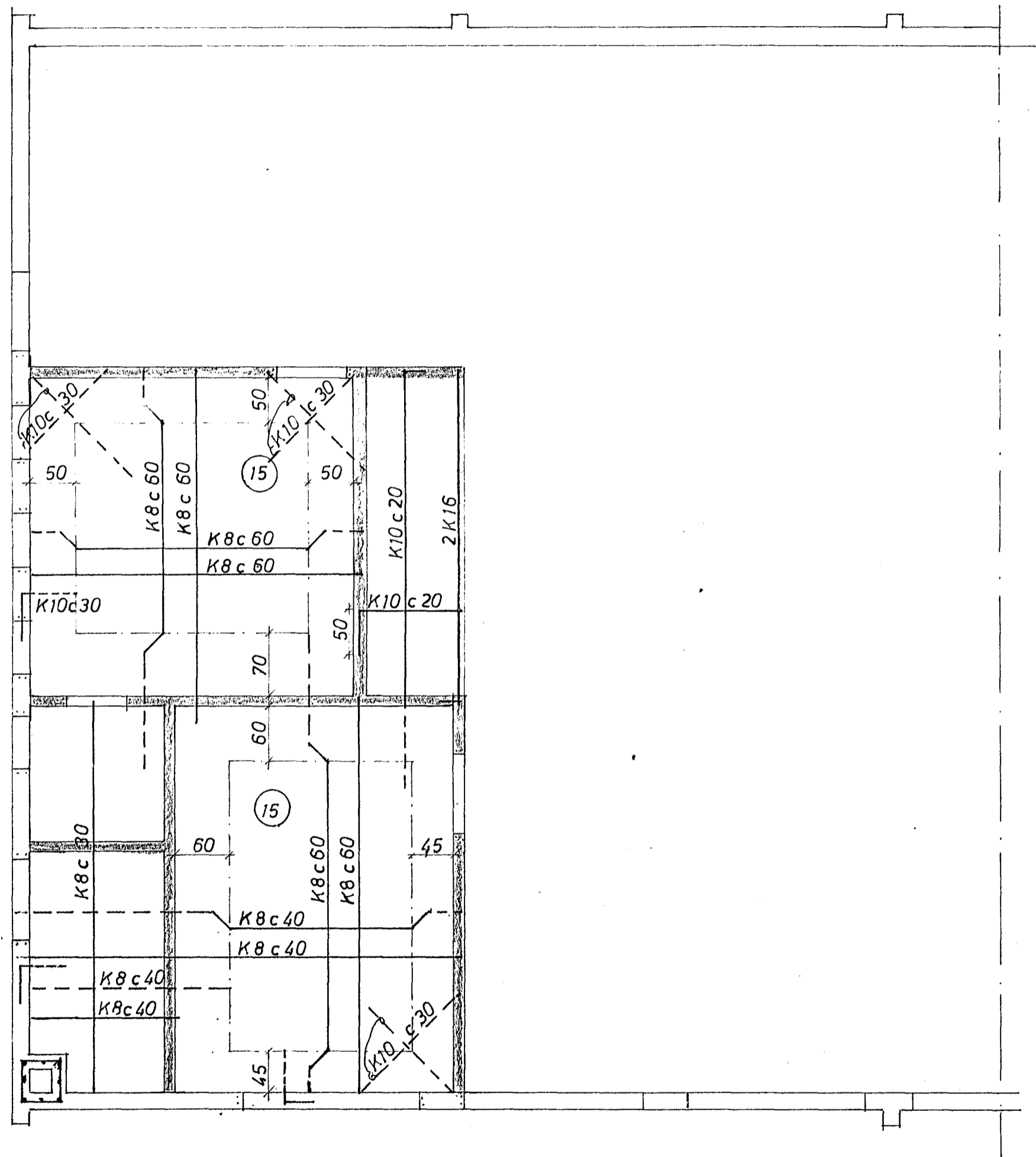
GRUNNMYND 1:50
